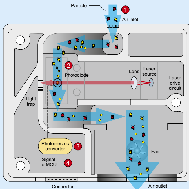
Rysunek 6. Zasada działania czujnika pyłów serii HPM115 firmy Honeywell [6]
