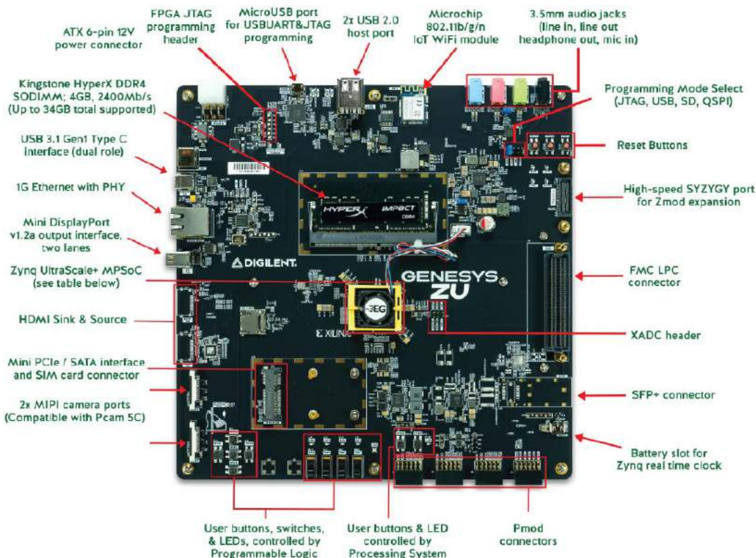
Fotografia 1. Wygląd zestawu Genesys ZU-3EG
