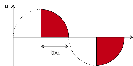
Rysunek 1. Idea regulacji fazowej
