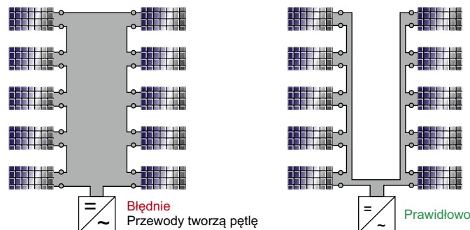
Rysunek 4. Dwa przypadki połączenia paneli na połaci dachowej
