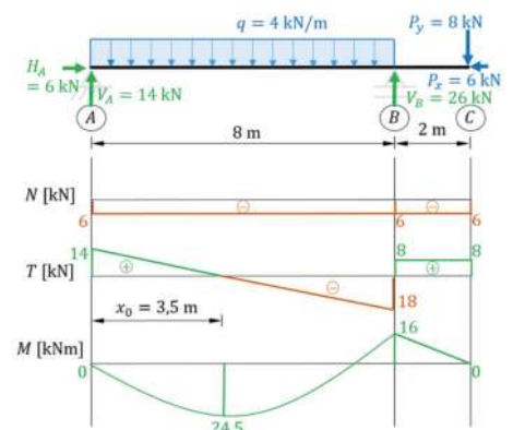
Rys. 12. Wykresy sił: osiowych, tnących, momentów zginających
