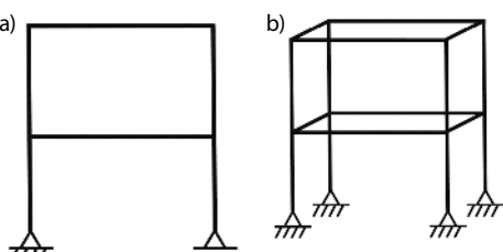
Rys. 2. Przykładowe schematy statyczne ram:
