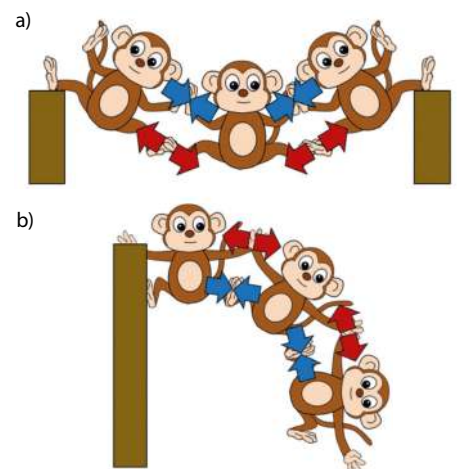
Rys. 13. Konwencje znakowania momentów zginających:
