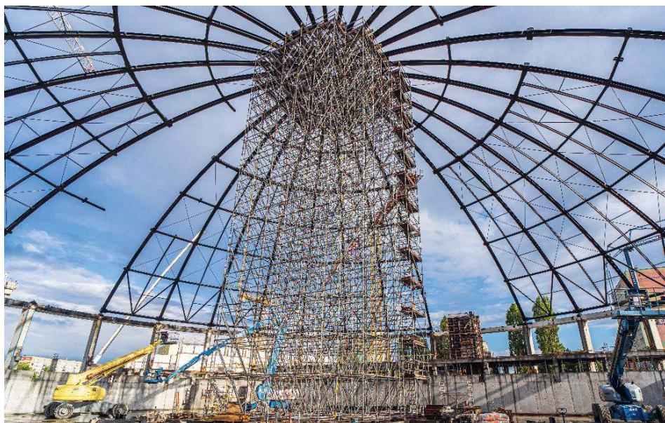
Fot. 2. Wieża o wysokości 27,5 m wykonana z rusztowania
