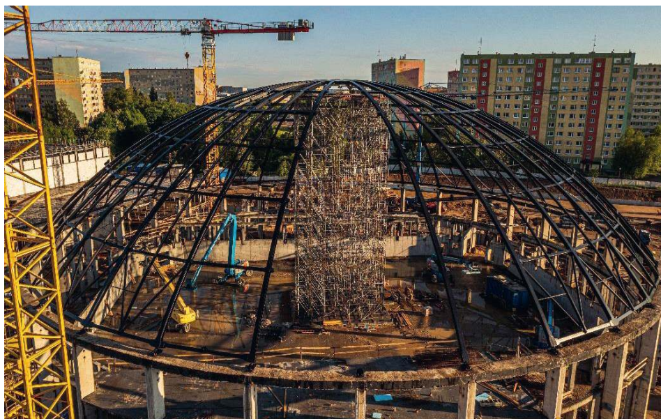
Fot. 1. Konstrukcja kopuły podczas scalania
