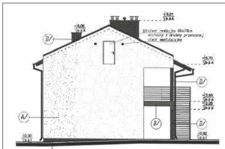
Elewacja południowa
