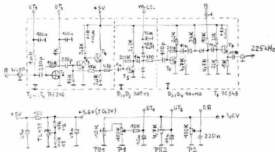
Rys. 1. Schemat wejściowego mnożnika dobroci
