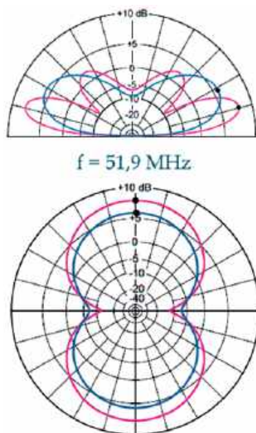
Rys. 3. Charakterystyki promieniowania anteny w płaszczyźnie pionowej i poziomej (linie niebieskie na wysokości 30 cm, fioletowe – 3 m)
