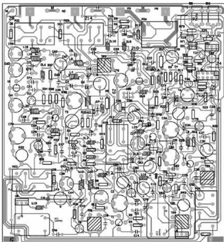
Rys. 3. Płytki transwertera
