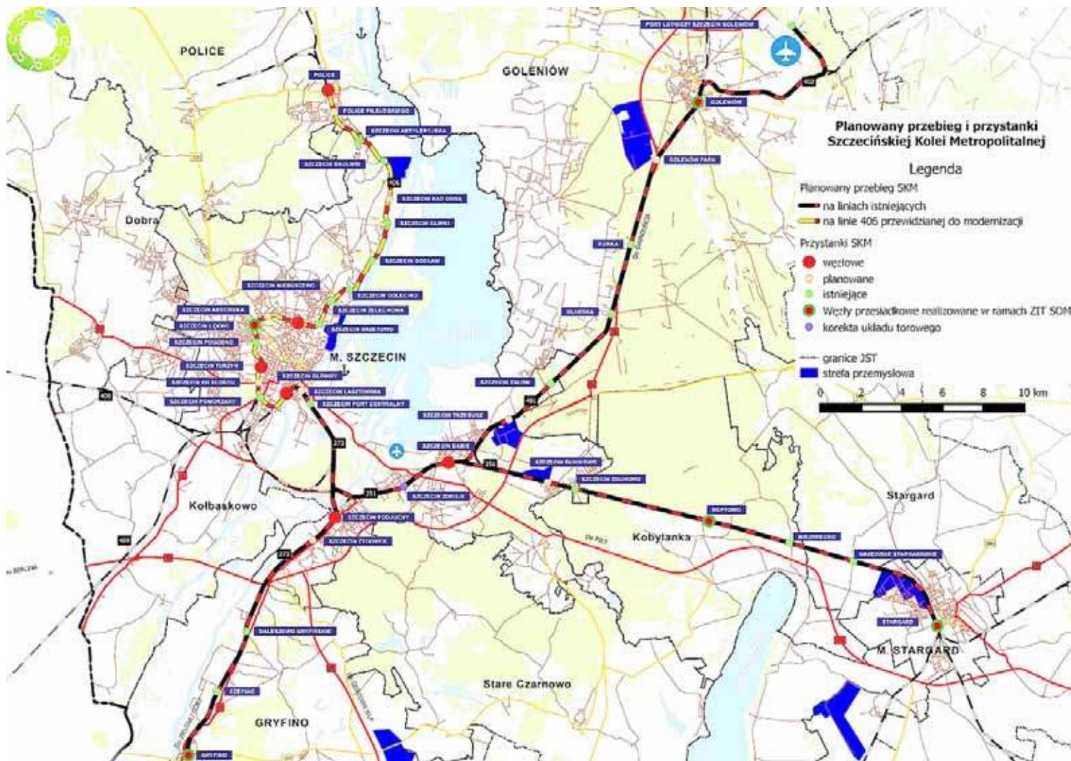
Planowany przebieg Szczecińskiej Kolei Metropolitalnej
