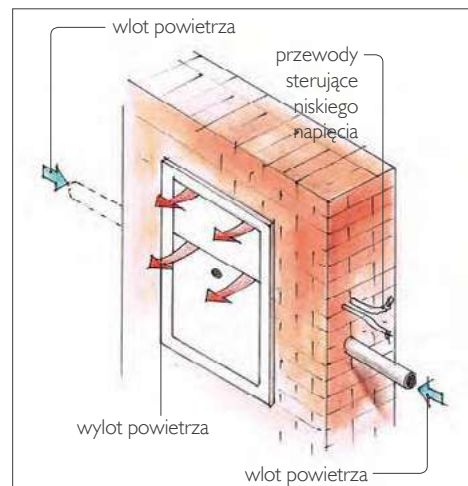
➌ Wydech powietrza przez szczeliny wokół drzwi szafki.
