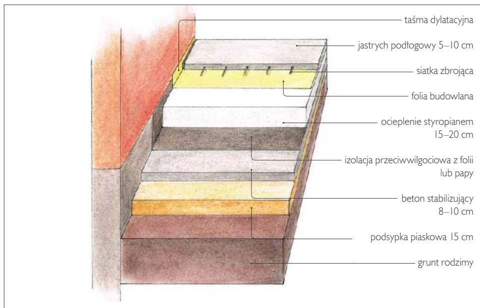
Podłoga na gruncie.
