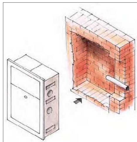
➋ Montaż podtynkowy.
