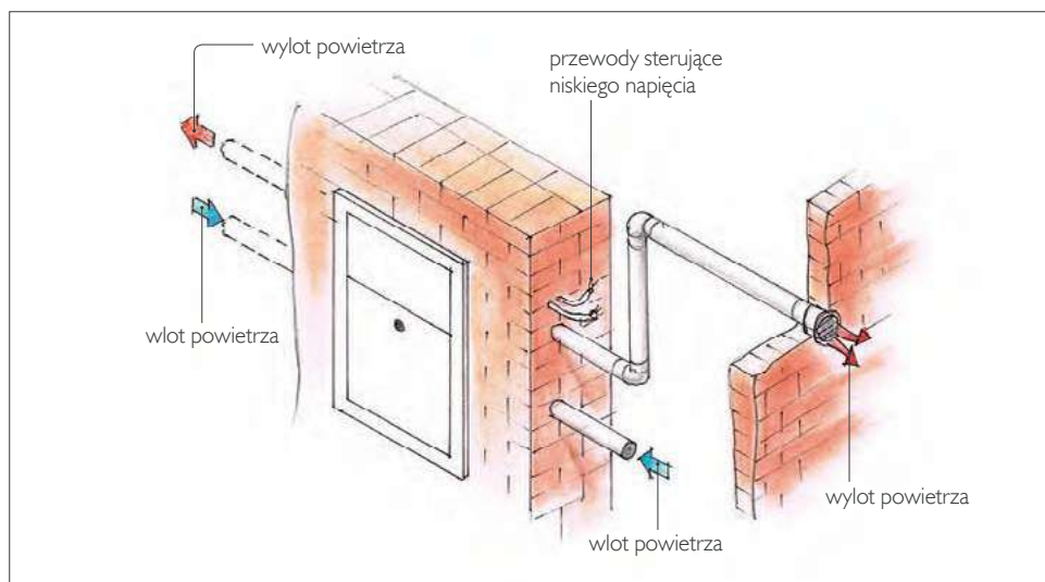
❶ Wydech powietrza na zewnątrz budynku.
