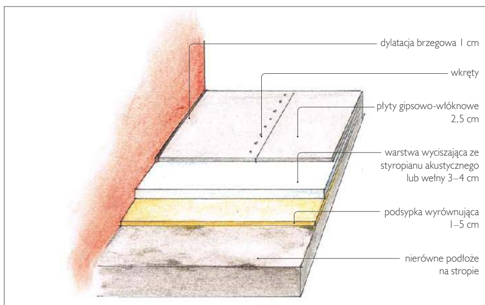
Podłoga na stropie żelbetowym.
