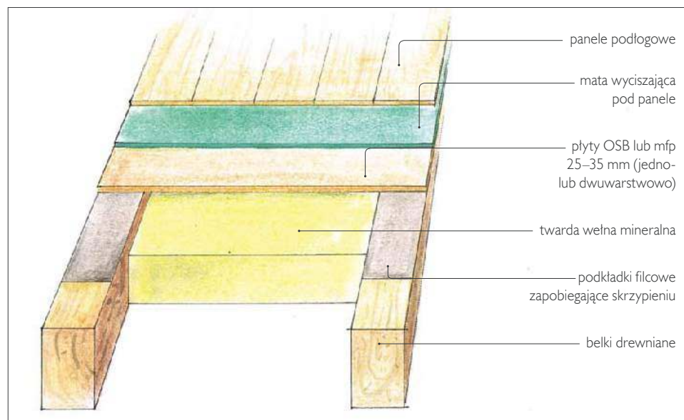
Podłoga na stropie drewnianym.
