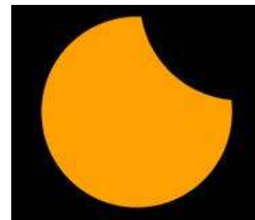
Symulacja tarczy Słońca podczas nadchodzącego zaćmienia
