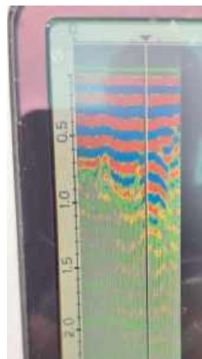
Eksperci ze Stowarzyszenia Wizna 1939 pomogli przebadac georadarem miejsce w którym, według opowieści dziedzica Szlubowskiego, zostali pochowani rozstrzelani przez Moskali powstańcy styczniowi. Udało się zidentyfikować miejsce, gdzie na przestrzeni około 2/3 metra struktura gruntu jest zaburzona, wyraźnie różni się od reszty badanego placu. Czy to oznacza grób? Na takie twierdzenie jest jeszcze za wcześnie
