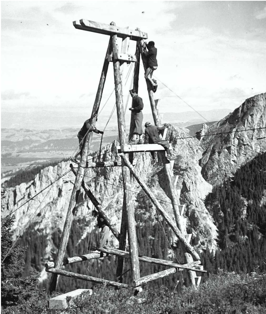
▲ Robotnicy budują drewnianą podporę pomocniczą kolejki transportowej. Niekiedy musieli pracować w ekstremalnych warunkach, przy silnym wietrze, na mrozie i w śniegach, 1935 rok
