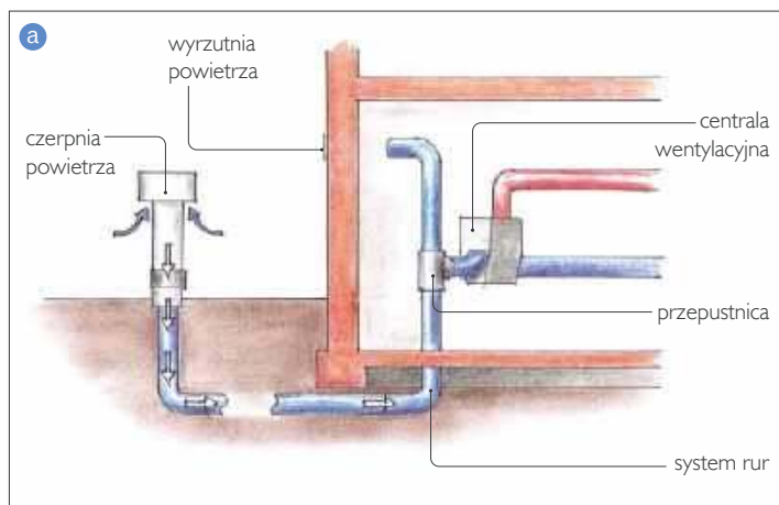
Gruntowy wymiennik ciepła rurowy (a), żwirowy (b).
