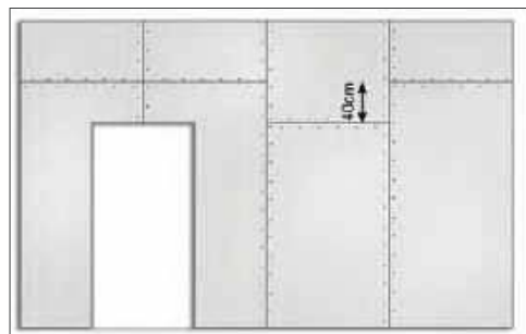
🔗 Miejsca łączeń płyt g-k w systemie lekkiej zabudowy powinny się odpowiednio mijać.
