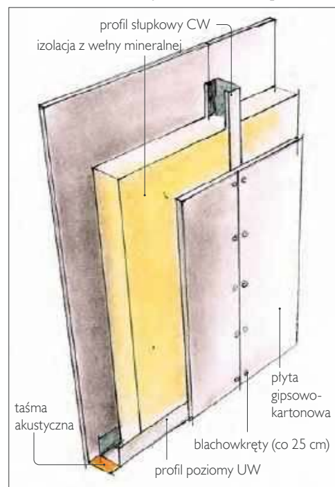
🔗 Ściana działowa z jednowarstwowym poszyciem z płyt g-k.
