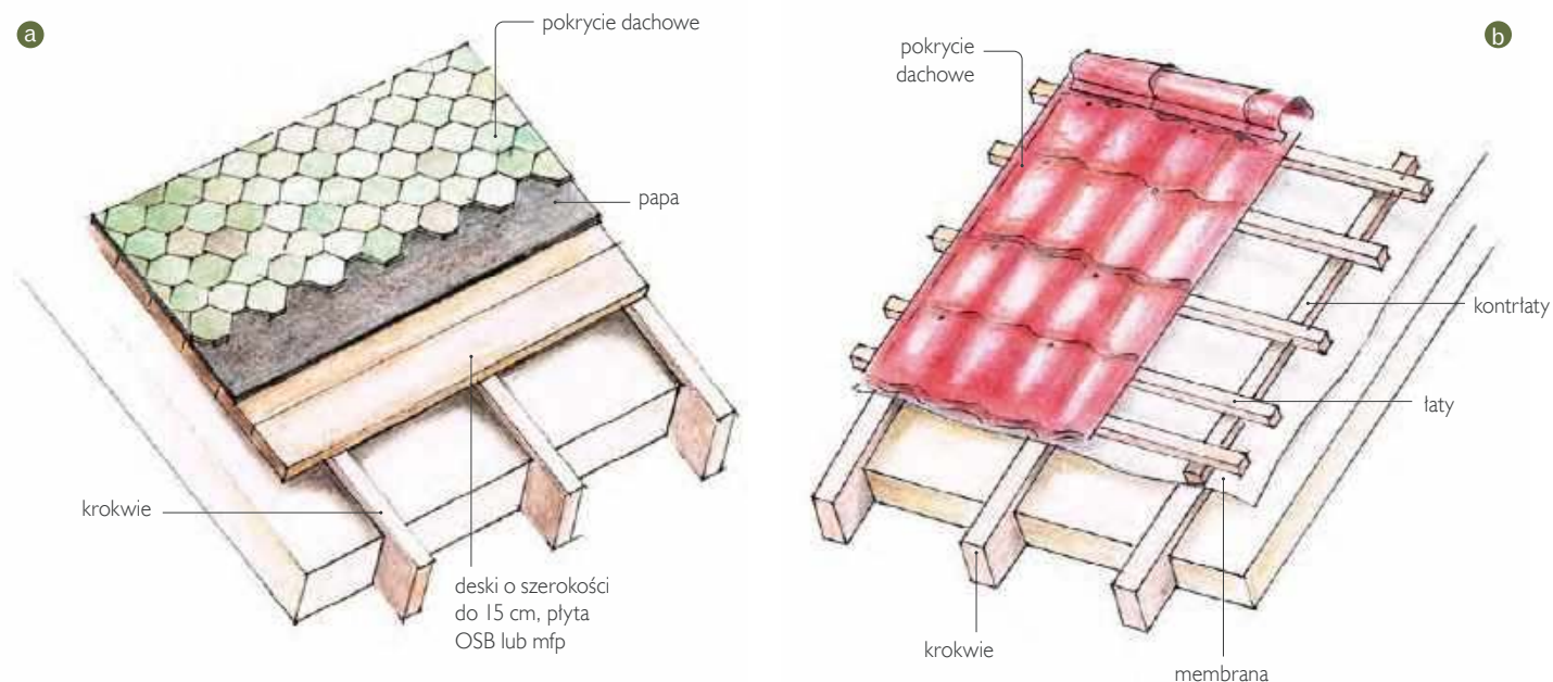
☞ Pokrycia dachowe wymagają podkładu. Może mieć on formę deskowania (a) lub ołacenia (b).
