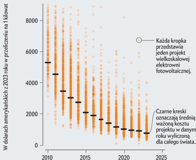
Średni koszt instalacji wielkoskalowego zestawu fotowoltaicznego na świecie
