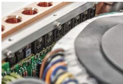
Tranzystory wyjściowe przykręcono bezpośrednio do miedzianych radiatorów.
