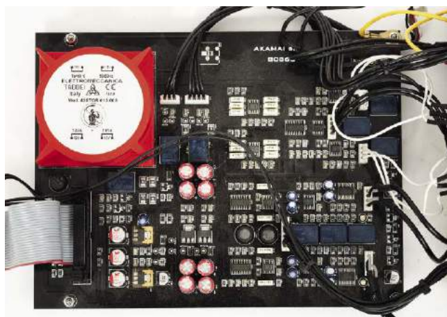
Niemal cały układ elektroniczny, włącznie z zasilaniem, zajmuje dużą płytkę drukowaną, ale gniazda podłączono już przewodami.
