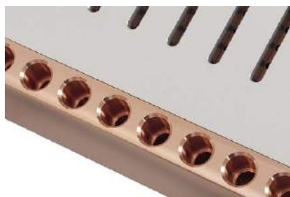
Główne radiatory wykonano z miedzianych bloków, pionowe otwory o zmiennych średnicach wspomagają przepływ powietrza zasysanego spod dolnej ścianki.
