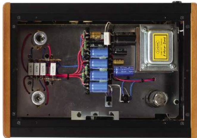
Układ wydaje się stosunkowo prosty, ale obecność lamp wymaga zastosowania starannie wyselekcjonowanych elementów.
