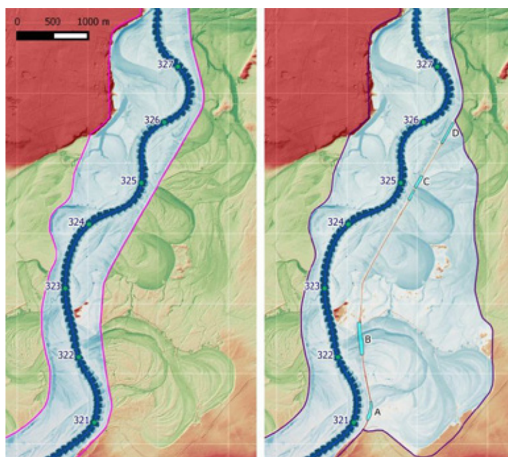
Profile głębokości korycie Odry wraz z zaznaczonymi obniżeniami wałowymi.
