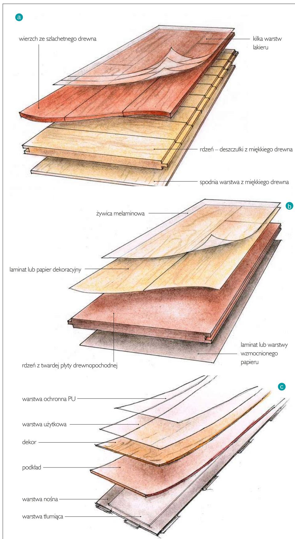
Warstwowa budowa panelu drewnianego (a) i laminowanego (b) i winylowego (c).
