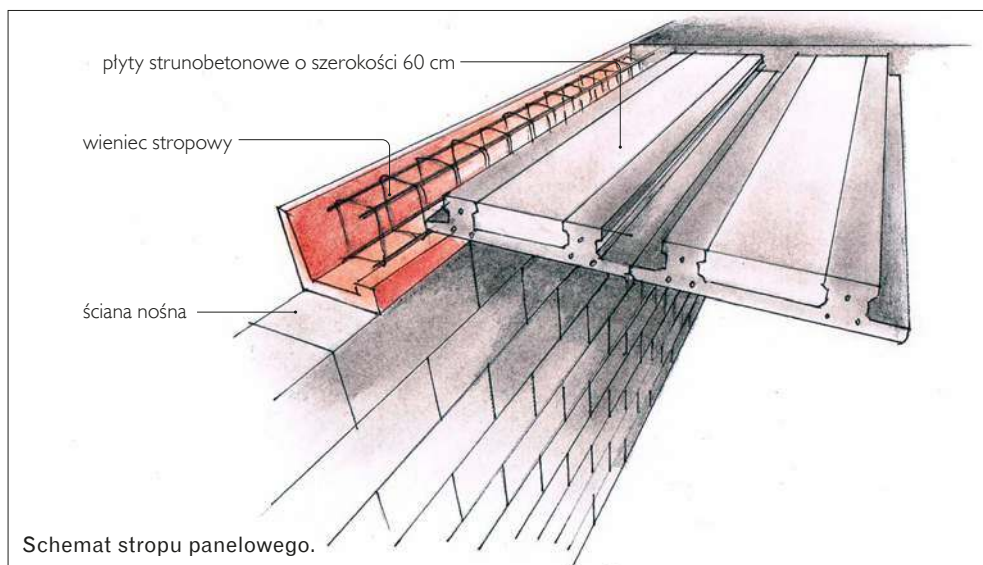
Strop z płyt prefabrykowanych kanałowych.
