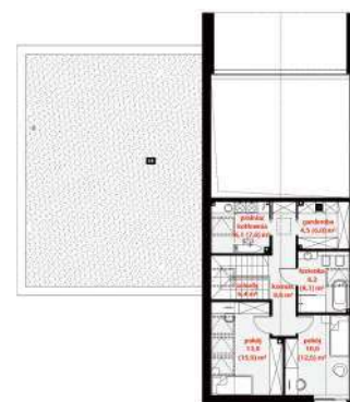
RZUT PODDASZA
