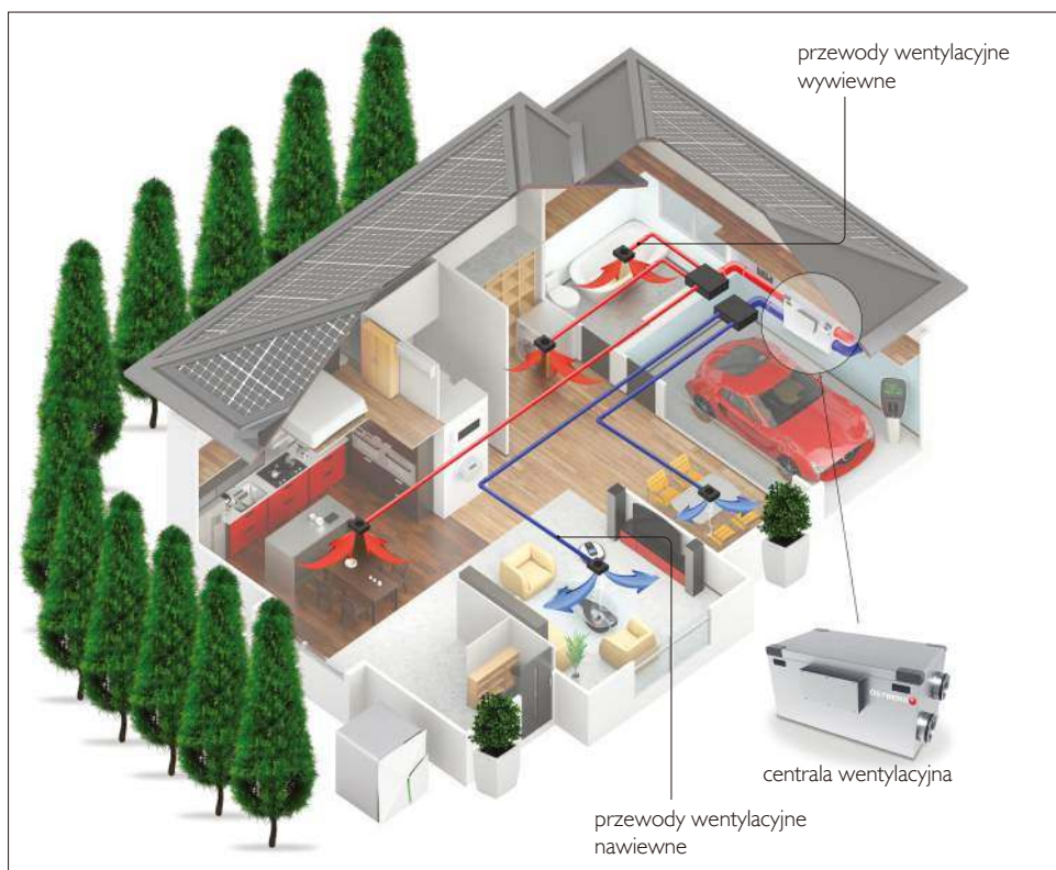
📌 Schemat wentylacji mechanicznej z rekuperacją. NEOVENT
