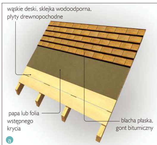
🔧 Pełne deskowanie (a) i ruszt z łat i kontrłat (b).
