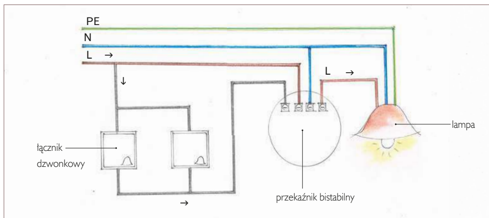
ⓘ Przełącznik bistabilny wraz z łącznikami dzwinkowymi.
