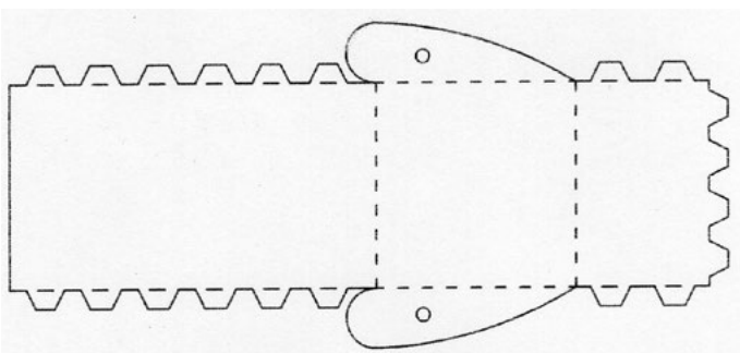
Rys. 7. Wzór do skopiowania na karton, wycięcia i sklejania płyty aerodynamicznej.
