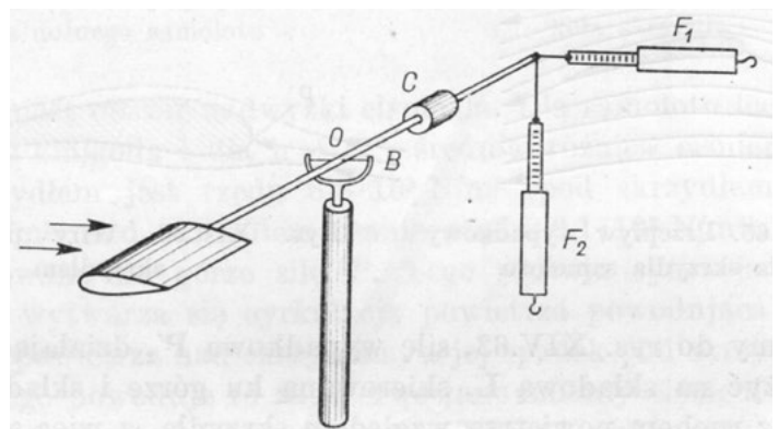
Rys. 5. Schemat wagi aerodynamicznej; O – os pionowa, B – os pozioma, C – ciężarek, F_1, F_2 – siłomierze do pomiaru siły oporu i siły nośnej, źródło [2].
