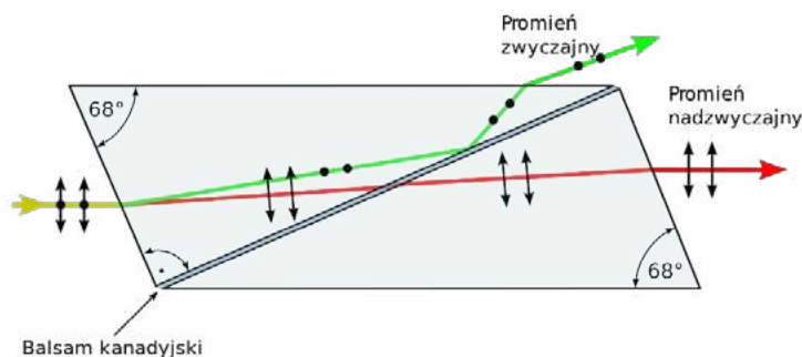
Rysunek 9. Bieg promieni w pryzmacie Nicol. Źródło: Autorstwo Cepheiden – File: Nicols_prism_DE.svg, CC BY-SA 3.0, https://commons.wikimedia.org/w/index.php?curid=31664530 [9].
