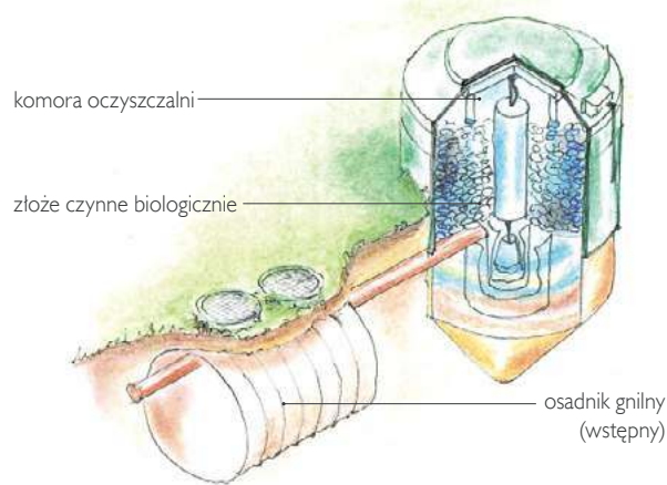
Wspólną cechą wszystkich oczyszczalni kompaktowych jest to, że cały proces zachodzi w kontrolowany sposób, wewnątrz urządzenia.
