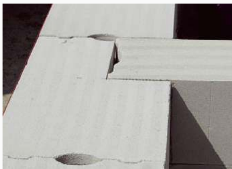
❗ Właściwe przemurzenie ściany nośnej z działową. SOLBET
