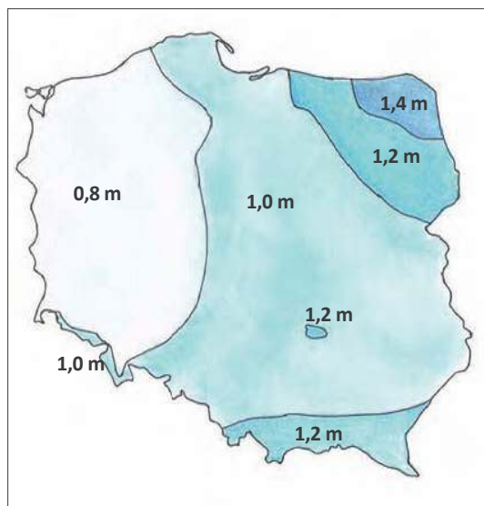
Strefy przemarzania gruntu w Polsce.
