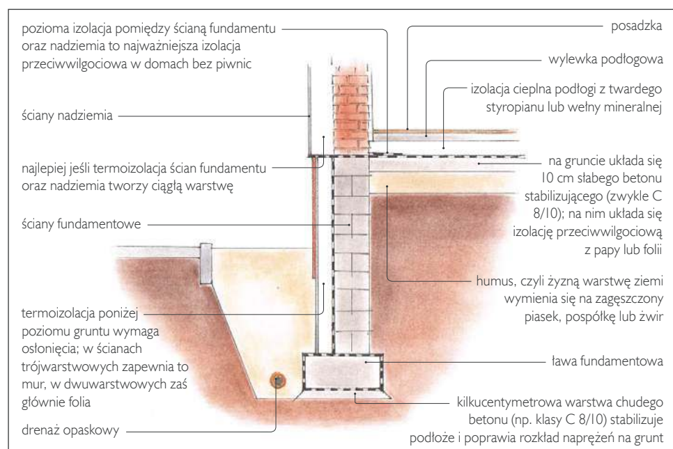
Schemat typowego fundamentu.
