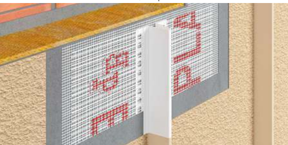
BP19 LISTWA PVC OZDOBNA „NA RABEK” Z SIATKĄ WRAZ Z ZASLEPKĄ SYSTEMOWĄ
