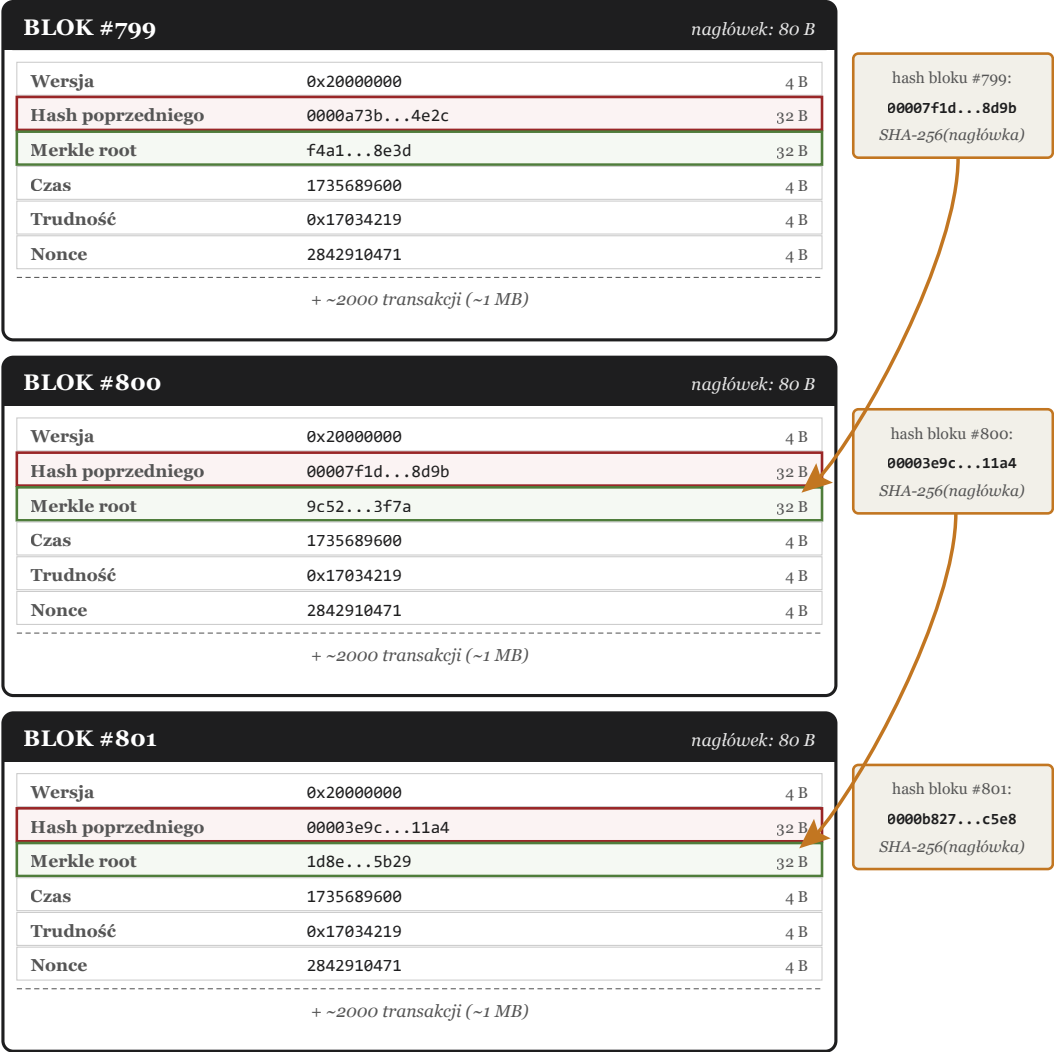
Rysunek 4. Trzy bloki w łańcuchu. Każdy z 6-polowym nagłówkiem. Hash każdego bloku jest wpisany w nagłówek następnego – to dlatego nazywa się to blockchain. Zmiana czegokolwiek w bloku 800 unieważnia wszystkie po nim
