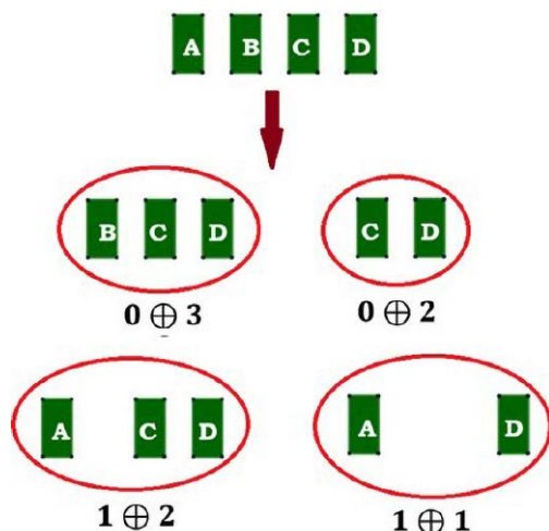
Rysunek 6. Diagram do obliczenia G(4)
