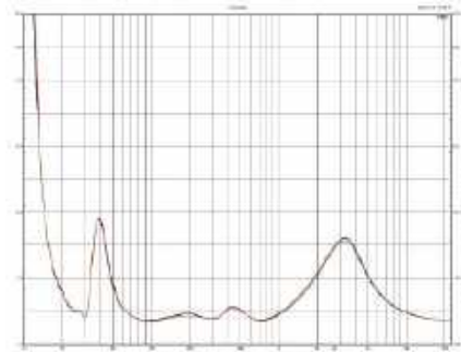
Rys. 3. Charakterystyka modułu impedancji 801 D4/801 D5
