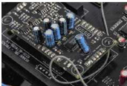
Przetwornik C/A to wciąż bardzo lubiany Burr Brown PCM1796.
