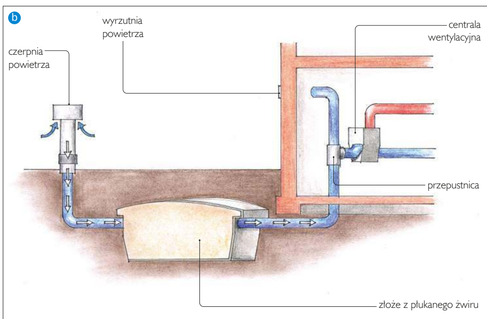
Gruntowy wymiennik ciepła rurowy (a), żwirowy (b).
