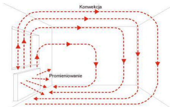
❶ Sposoby oddawania ciepła przez grzejnik ścienny.
