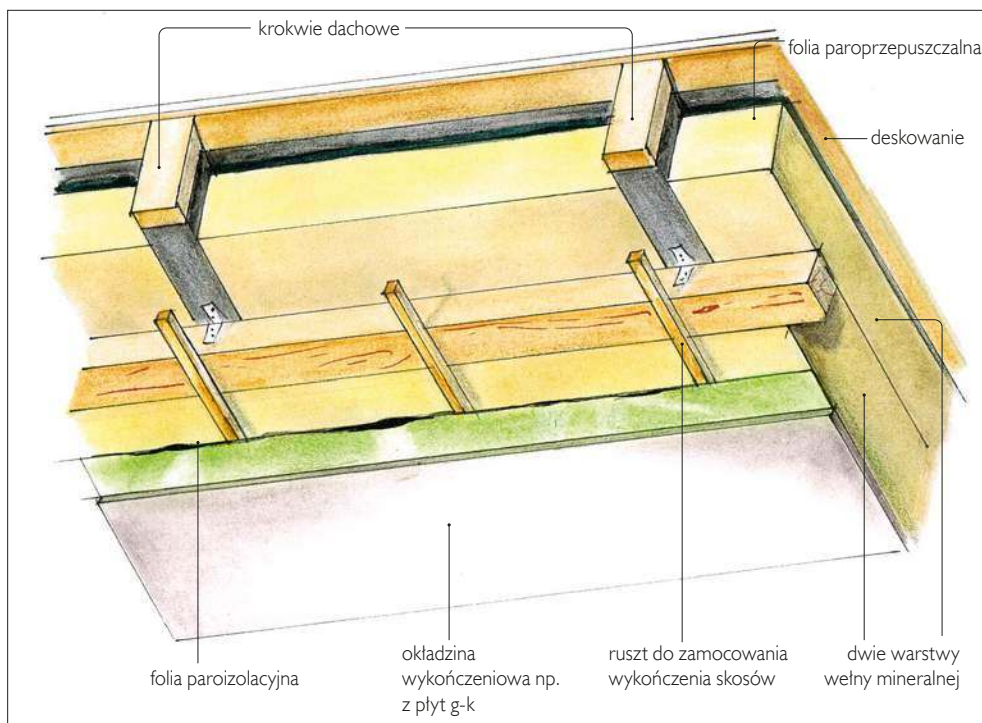
❗ Schemat ocieplenia dachu skośnego wełną mineralną.
