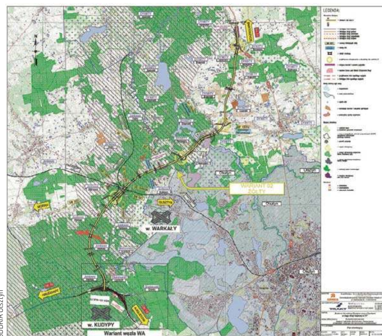
Plan północnej obwodnicy Olsztyna
