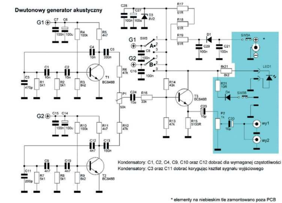
Rys. 3. Schemat ideowy generatora dwutonowego m.cz. wg SP4IRX
