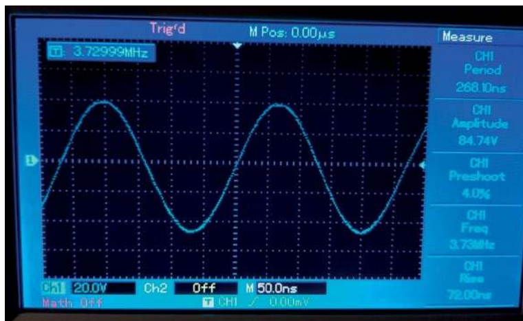
Przebieg napięcia wyjściowego wzmacniacza mocy podczas prób
