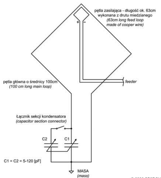
Rys. 1. Schemat konstrukcji anteny
