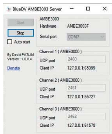
Rys. 3. Konfiguracja oprogramowania serwera AMBE3003
