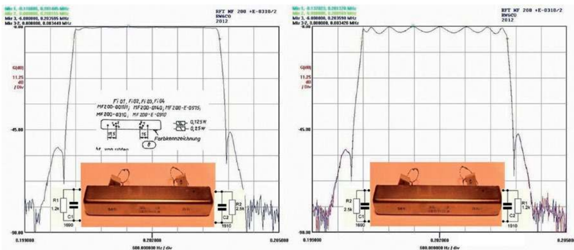
Rys. 1. Charakterystyka filtra MF 200 + E-0310/2
