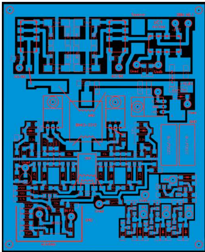
Rys. 1. Widok projektu płytki z układem zasilania, wzmacniacza mocy, filtrów dolnoprzepustowych i układu sterującego załączaniem przekazników
