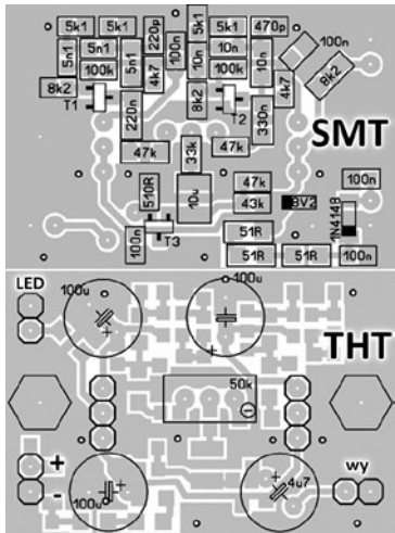
Rys. 5. Rozmieszczenie elementów na płycie drukowanej generatora
