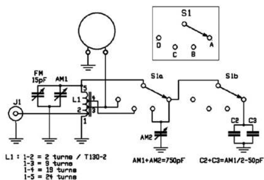
Rys. 6. Schemat anteny pętlowej 160-10 m
