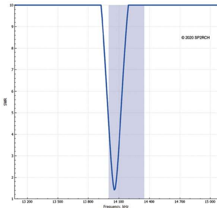
Rys. 2. Wykres charakterystyki SWR w paśmie 20 m
