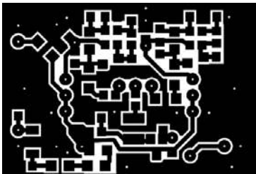
Rys. 4. PCB generatora (lustrzane odbicie)
