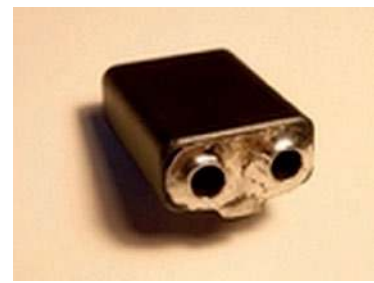
Transformator Tr2 z uzwojeniem pierwotnym w postaci rurek
