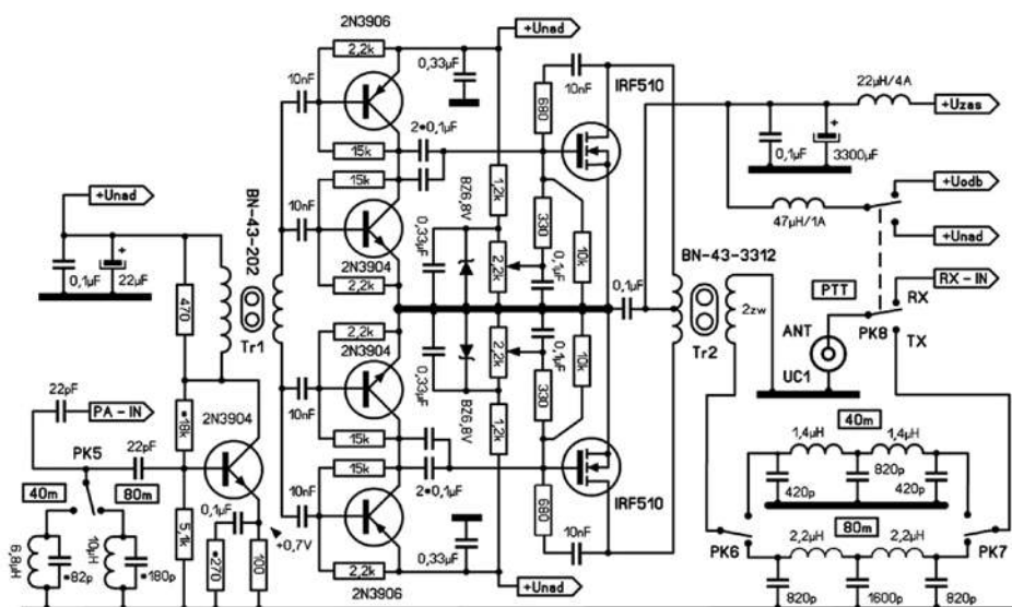
Rys. 4. Schemat wzmacniacza mocy w.cz. z obwodami selektywnymi na wejściu i filtrami dolnoprzepustowymi na wyjściu
