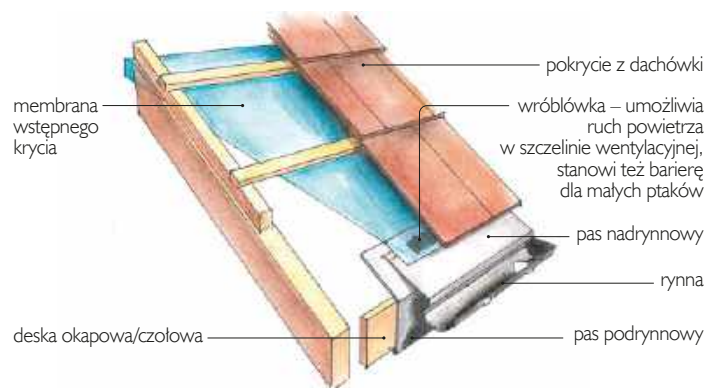
Obróbki okapu.
