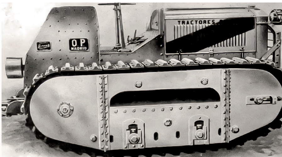
▲ Traktor Benach OP no 4 (OP czyli Obras Públicas, roboty publiczne). Czwarty model traktora, dzięki któremu zakłady odniosły olbrzymi komercyjny sukces. Z warsztatów produkujących maszyny rolnicze zakłady przekształciły się w producenta pojazdów dla wojska.
