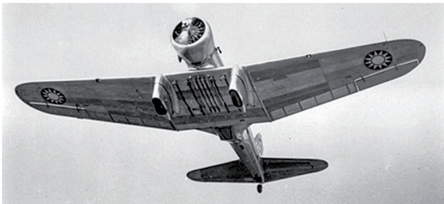
▲ Northrop Gamma 2E krótko po starcie. Widać wyrzutniki bombowe pod centroptatem.
