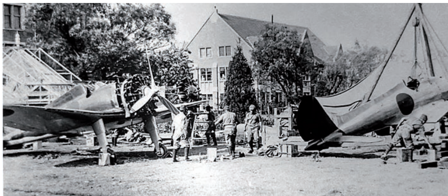
▲ Samoloty myśliwskie Mitsubishi A5M1 i A5M2 Ko na lotnisku Kuang-Ta w Szanghaju około 10 września 1937 roku. Chociaż cenzor usunął oznaczenia na ogonach, wydaje się, że myśliwce należą do 13. Kōkūtai, która została tu przebazowana 9 września 1937 roku.
