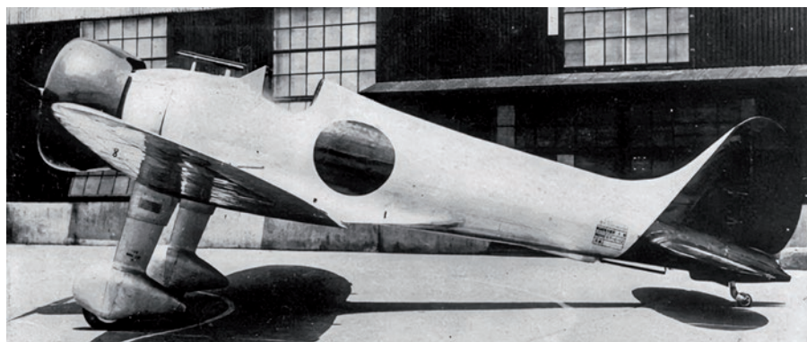
▲ Mitsubishi A5M1 w widoku z lewej strony. Pierwszą walkę myśliwce tego typu stoczyły 4 września 1937 roku i szybko udowodniły swą techniczną przewagę nad chińskimi myśliwcami.
