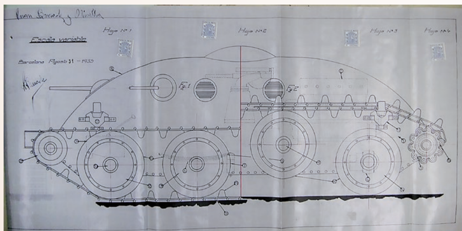
▲ Projekt czołgu opracowany przez inż. Joan Benach i Olivella w 1935 roku. Zwracają uwagę duże koła jezdne oraz sposób transportu gąsienic w momencie, gdy pojazd miał poruszać się na kołach.
