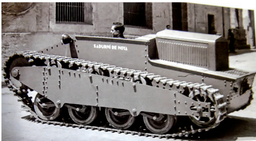
▲ Zmodyfikowany ciągnik gąsienicowy Sadurni miał węższy kadłub (brak sponsonów nad gąsienicami), przedział silnikowy oddzielony był od przedziału załogi przegrodą (był tam zainstalowany zbiornik paliwa). Po próbach zdecydowano się na zamontowanie osłon przeciwpiaśkowych.
