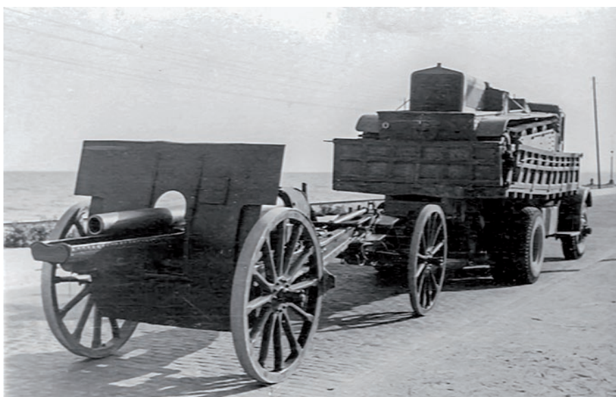
▲ Ciągnik Sadurni przewożony samochodem FWD M-10. Pojazd ma już zainstalowane osłony przeciwpiaśkowe z boku kadłuba.
