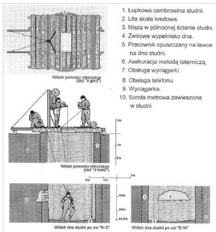
Schematyczne wyobrażenie pomostu roboczego i prowadzenia zjazdów na dno studni podczas badań penetracyjnych 5-8 grudnia 1996 r., rys. Karol E. Natkański.
