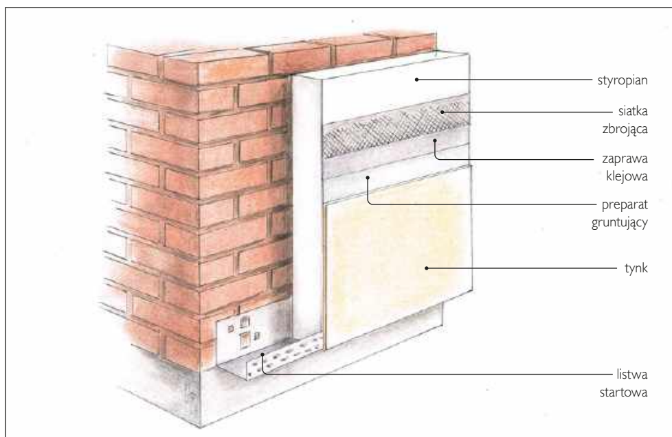
🔑 Ściana ocieplona metodą lekką moką.
