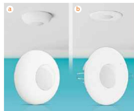
❗ Sufitowe czujki podczerwieni – nawierzchniowa do montażu do każdego typu powierzchni (a) i wpuszczana, przeznaczona do sufitów podwieszanych i z płyt g-k (b). Czujki zalecane są do pomieszczeń z przeszkleńmi lub nietypowym układem ścian czy wysokich mebli, które mogą ograniczać pole detekcji. SATEL
