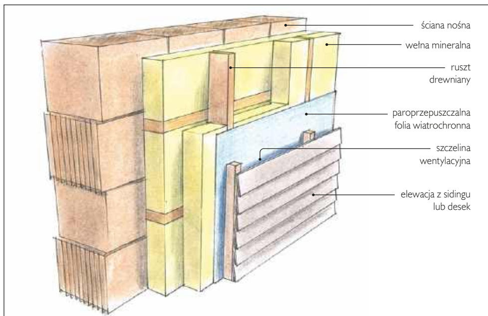
🔑 Ściana ocieplona metodą lekką suchą.
