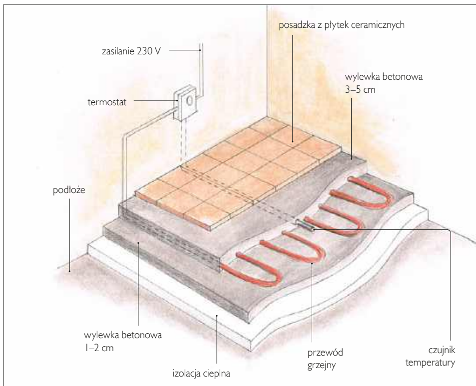
❗ Schemat elektrycznego ogrzewania podłogowego. Jego projekt dobrze jest zlecić doświadczonemu fachowcowi, który uwzględni zapotrzebowanie cieplne budynku, a także parametry techniczne zastosowanych materiałów instalacyjnych.
