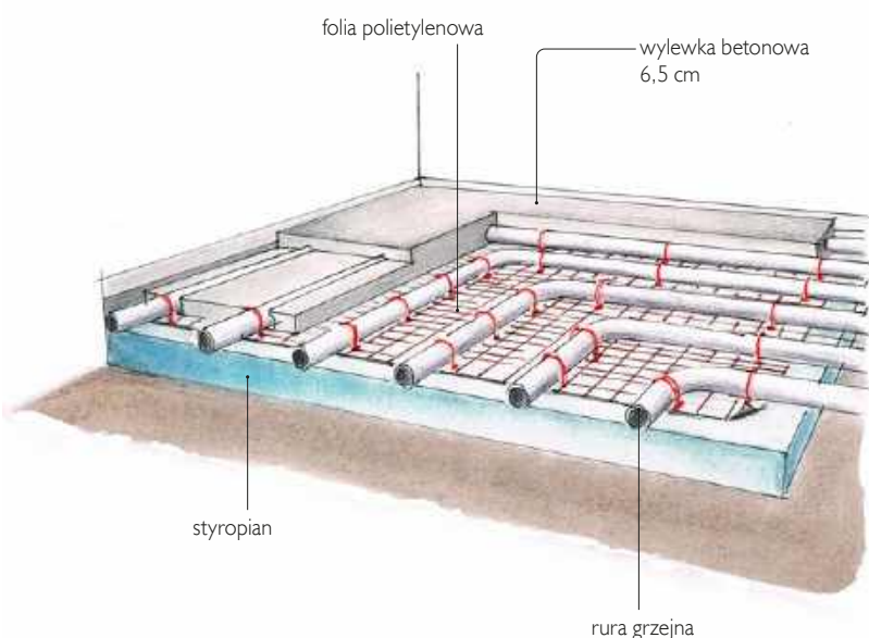
🔧 Sposób wykonania ogrzewania podłogowego w wersji wodnej.
