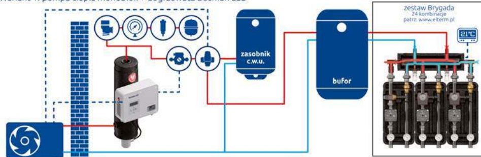
Wariant 1: pompa ciepła monoblok + dogrzewacz Bosman LED
