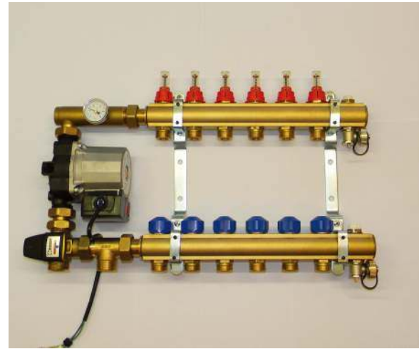
➡ Układ mieszający służy do połączenia instalacji grzejników ściennych z podłogówką. KISAN
