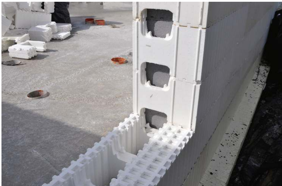
📍 Wykonane z kształtek styropianowych ściany mają bardzo dobre parametry termoizolacyjne, bo żelbetowy rdzeń jest z obu stron osłonięty ociepleniem. IZODOM2000
