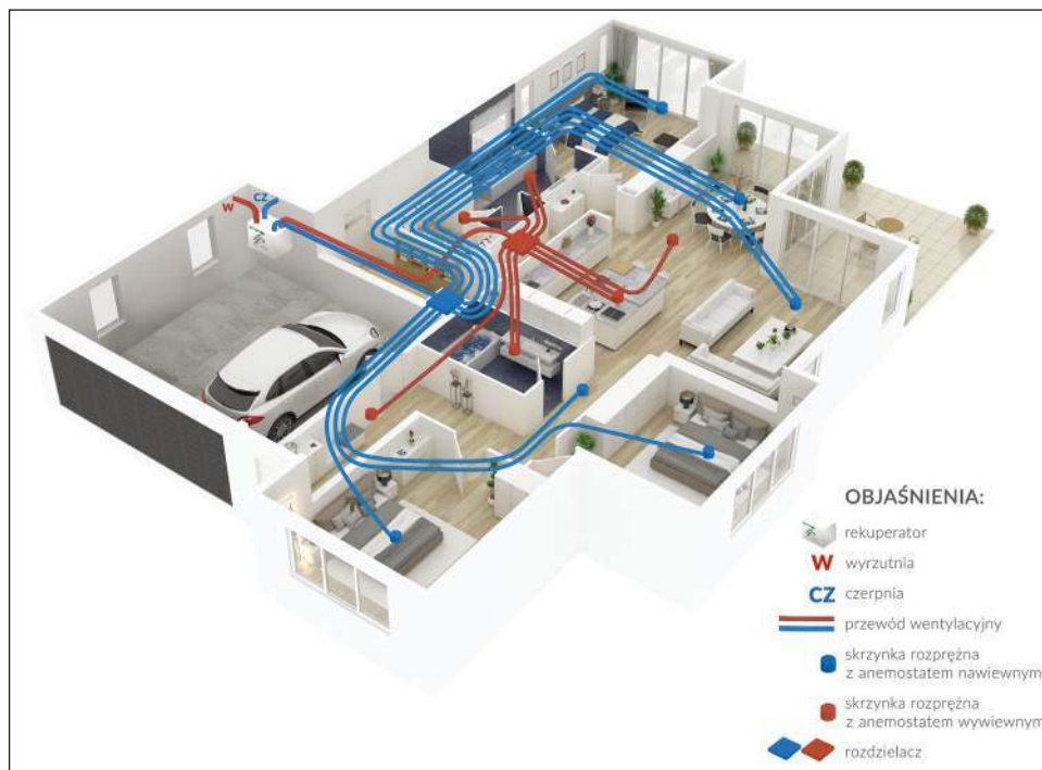
Schemat rozplanowania poszczególnych elementów wentylacji z odzyskiem ciepła. TOPVAC
