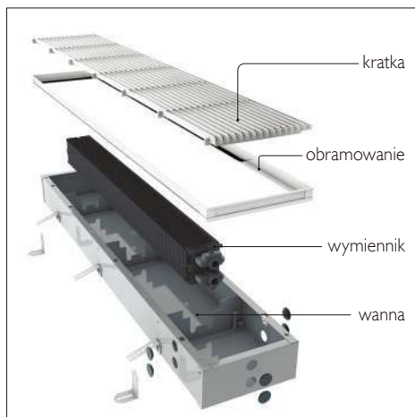
Poszczególne elementy grzejnika kanałowego. JAGA
