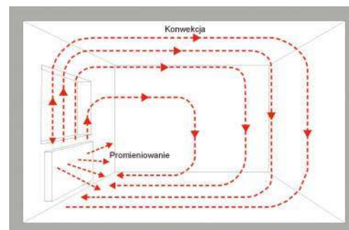
🔥 Sposoby oddawania ciepła przez grzejnik.
