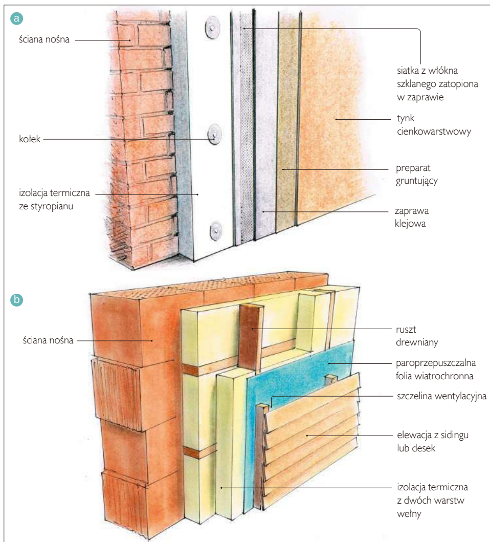
Ściana ocieplona metodą lekką mokrą (a) i metodą lekką suchą (b).
