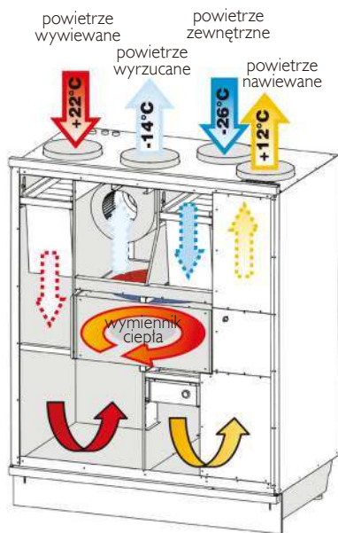
Zasada działania centrali z rekuperatorem. IGLOTECH
