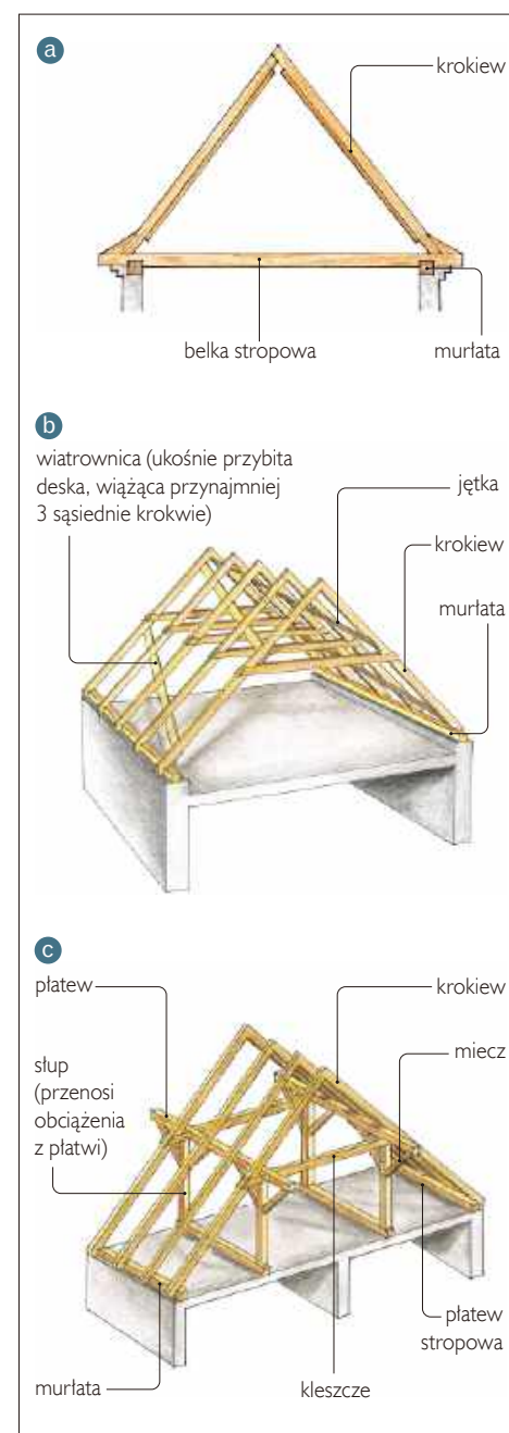
🔧 Tradycyjna więzba dachowa: krokwiowa (a), krokwiowo-jętkowa (b), płatwiwo-kleszczowa (c).
