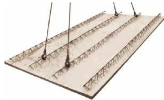
Strop typu filigran składa się ze zbrojonych płyt żelbetowych, przygotowywanych w fabryce. LEIER
