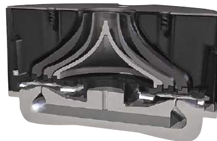
Klipsch dołożył wielką tubę i soczewkę akustyczną w formie kratki wentylatora.
