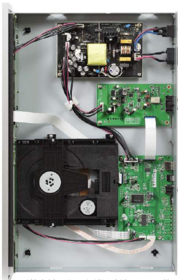
Układ elektroniczny CD350 podzielono na trzy główne moduły – zasilacz, odtwarzacz (płyty i plików) oraz przetwornik C/A.
