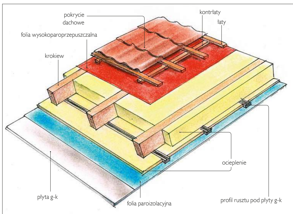
❸ Folie izolacyjne w konstrukcji dachu.
