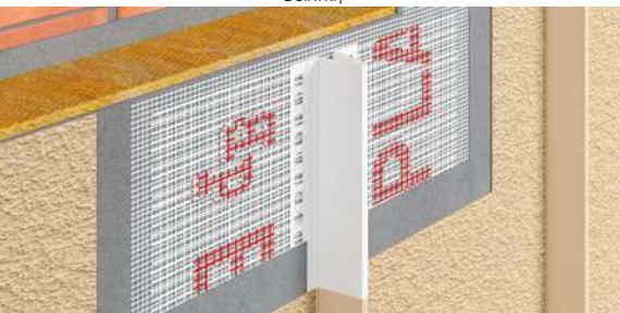
BP19 LISTWA PVC OZDOBNĄ „NA RABEK” Z SIATKĄ WRAZ Z ZASLEPKĄ SYSTEMOWĄ
