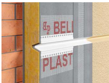
📌 Listwa z PVC do boniowania trójkątna – rąbek wklęsły. BELLA PLAST
