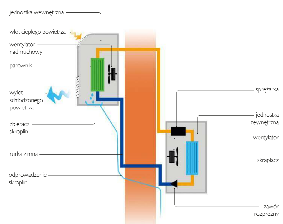
🔗 Schemat budowy klimatyzatora.
