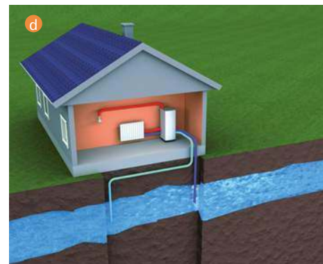
➦ Pompa może czerpać ciepło z – powietrza (a); gruntu z sondami pionowymi (b); gruntu z kolektorem poziomym (c); wód podziemnych (d). DANFOSS
