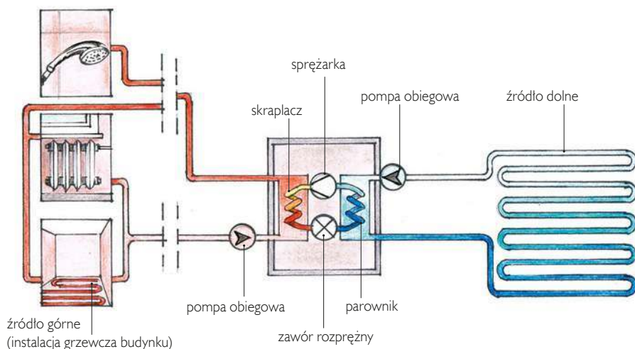
🔧 Zasada działania pompy ciepła.
