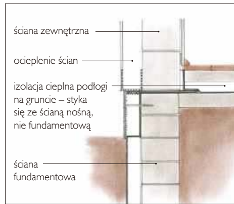
🔧 Prawidłowe połączenie izolacji cieplnej ściany fundamentowej, zewnętrznej i podłogi na gruncie.
