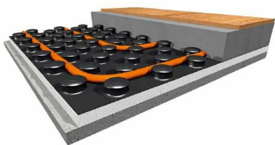
Płyta systemowa z wypustkami, pomiędzy którymi umieszcza się rurki grzewcze. Zastosowanie takiego rozwiązania pozwala przyspieszyć montaż i – dzięki cieńszej warstwie jastrychu – zmniejszyć ciężar podłogi. PURMO
