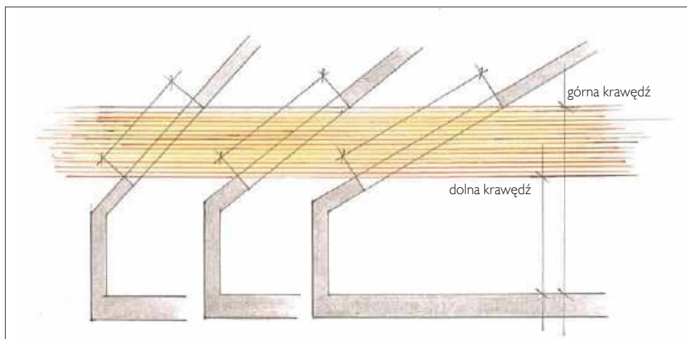
🔗 Im mniejszy jest spadek dachu, tym dłuższe powinno być okno, jeżeli jego górna krawędź ma być na tej samej wysokości.
