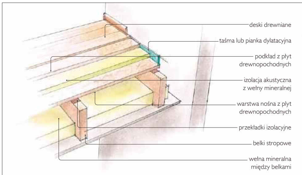
Schemat podłogi na stropie drewnianym.
