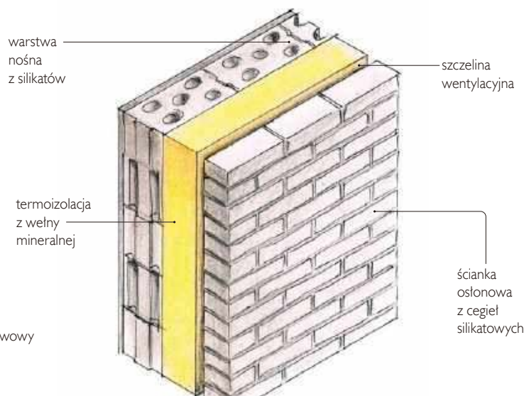
➤ Ściana trójwarstwowa.
