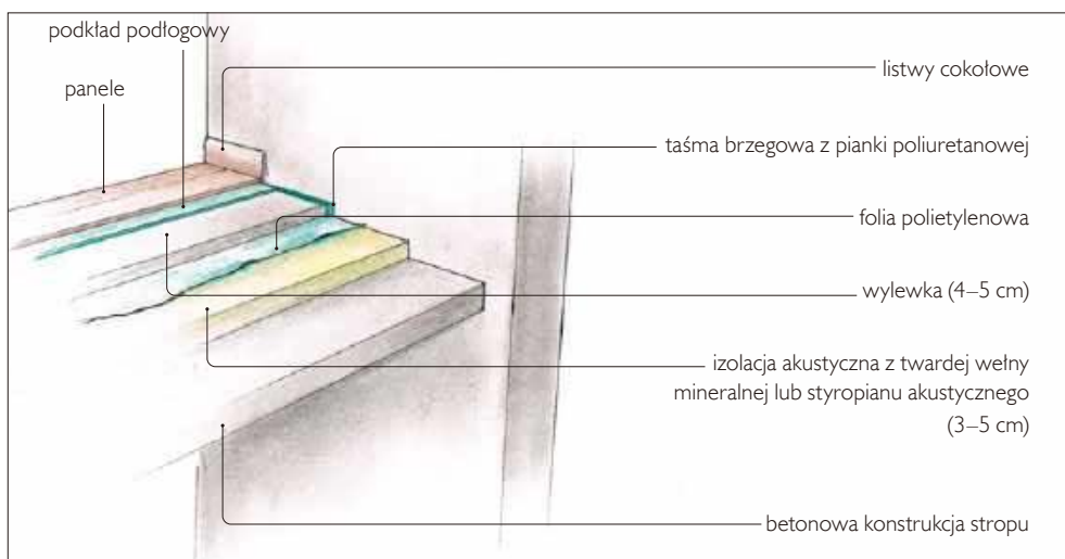
🔧 Warstwy podłogi na stropie żelbetowym.
