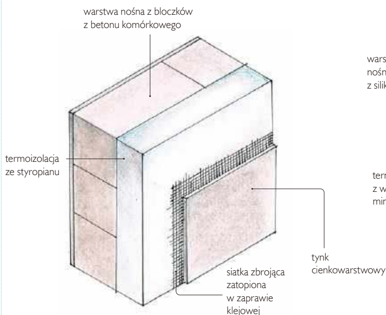
➤ Ściana dwuwarstwowa ocieplona metodą lekką mokrą.
