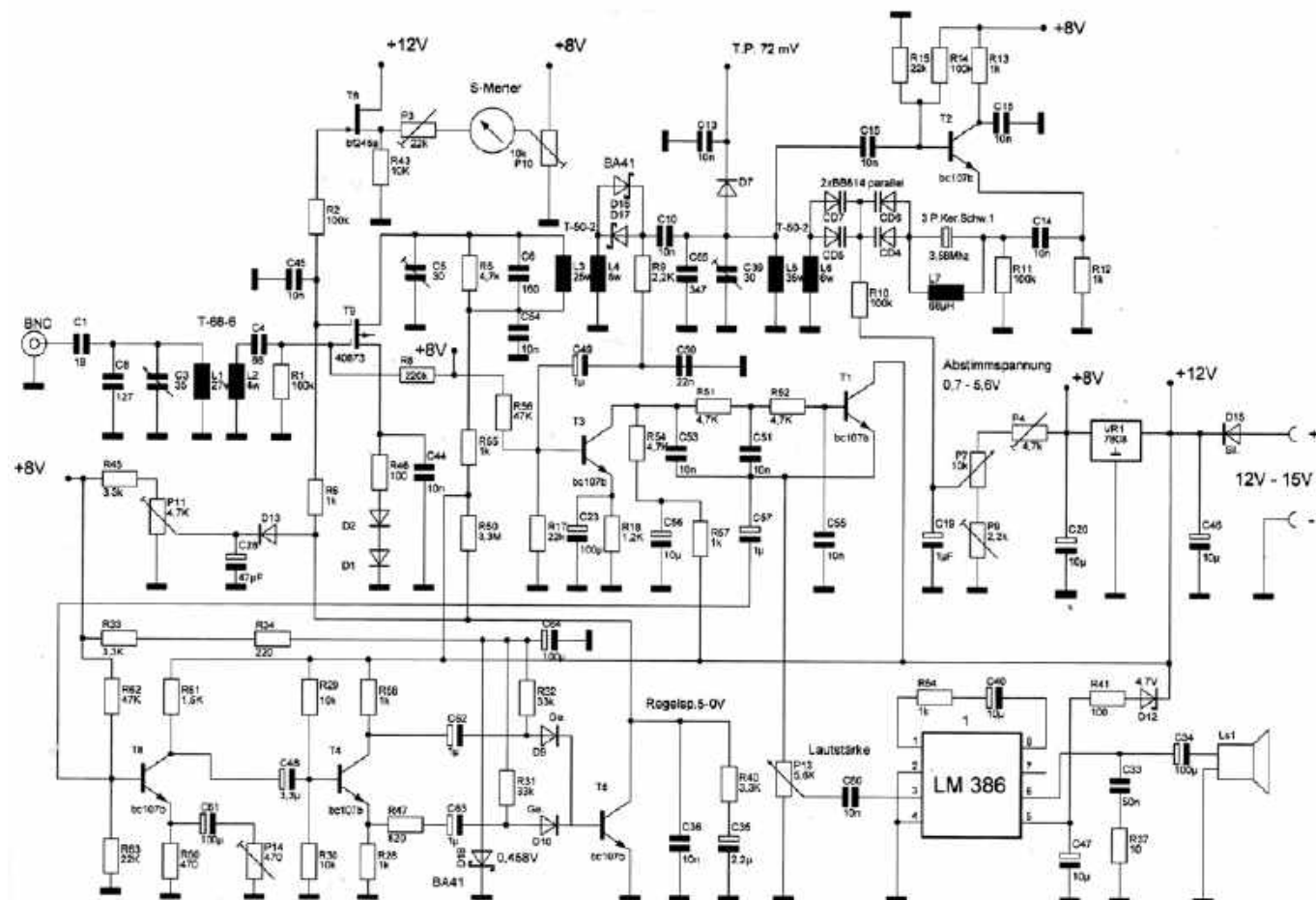
Rys. 1. Schemat ideowy odbiornika DC 40 m
