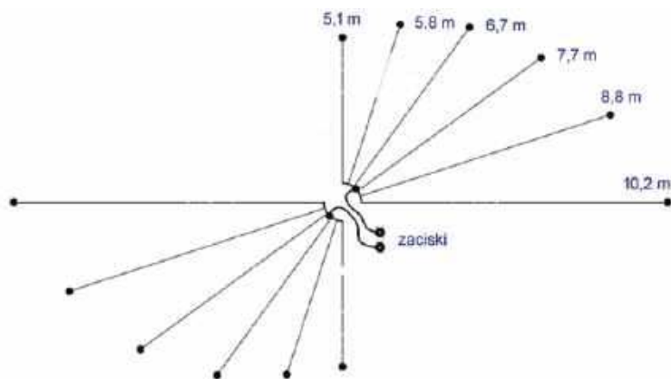
Rys. 3. Konstrukcja anteny wachlarzowej na pasma od 40 m wzwyż. Kąty pomiędzy dipolami wynoszą 18 stopni. Na rysunku podane są długości połówek dipoli
