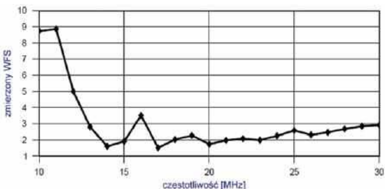
Rys. 2. Zmierzony przebieg WFS anteny na pasma 20–10 m dla systemu 50-omowego. Wyraźnie widoczny jest górnoprzepustowy charakter anteny
