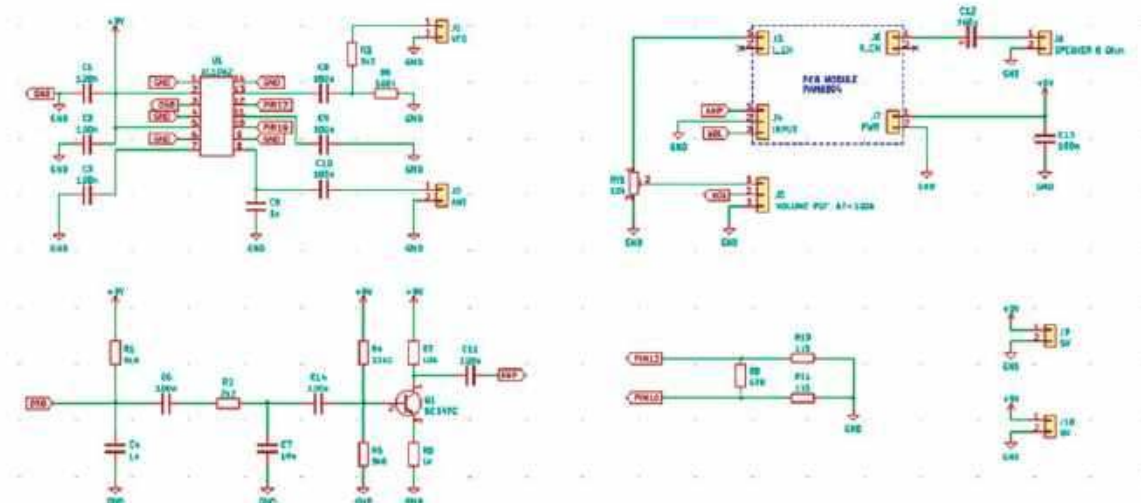
Rys. 4. Schemat układu odbiornika homodynowego
