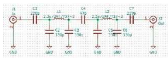
Rys. 1. Schemat filtra pasmowego
