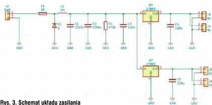
Rys. 3. Schemat układu zasilania
