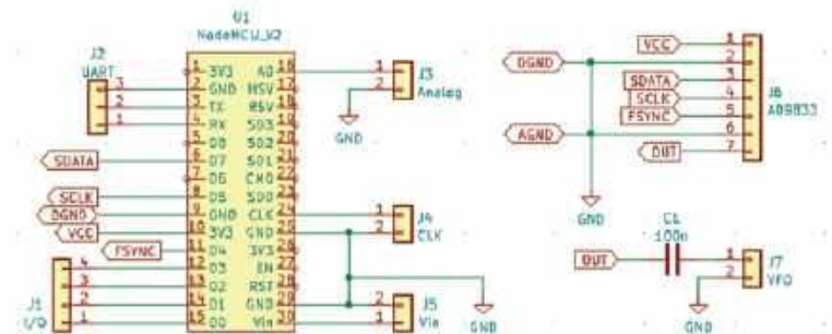
Rys. 2. Schemat przestrajanego generatora VFO
