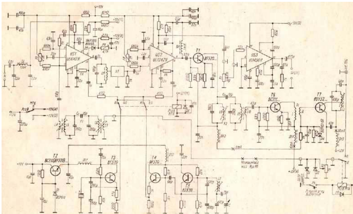
Rys.1 Schemat elektryczny minitranscevera Bartek z „Radioelektronika” 4–5/82
