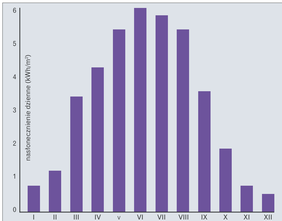
☛ Nasłonecznienie dzienne 1 m 2 powierzchni – płaszczyzna o nachyleniu 45° (dane dla Warszawy).
