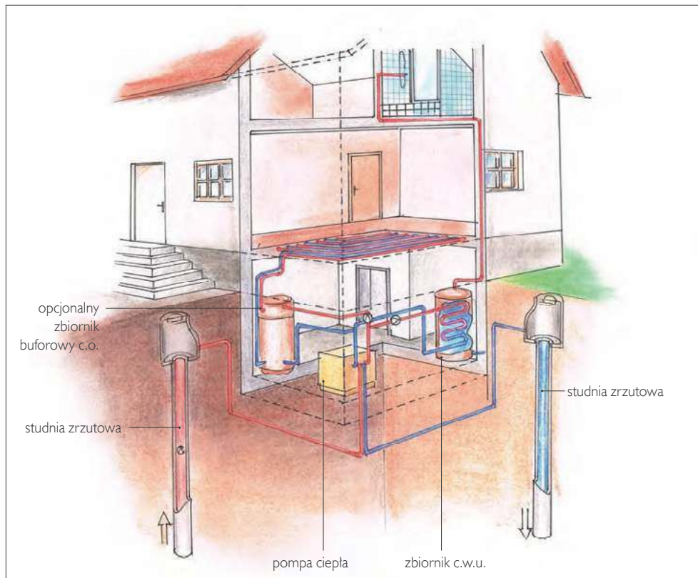
❶ Dwie studnie do wykorzystania wód podziemnych.
