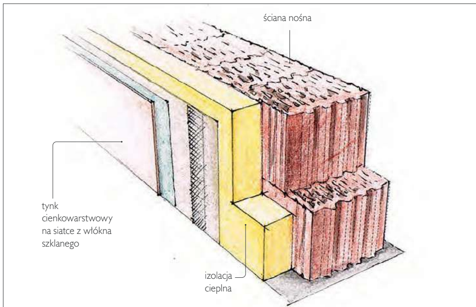
Ściana dwuwarstwowa ocieplona metodą lekką mokłą.
