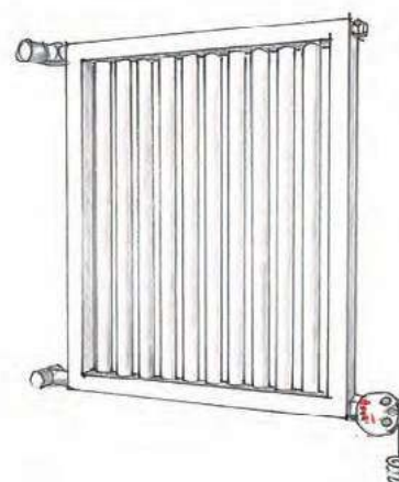
Rys. 5 Podłączenie poziome grzałki dopuszczalne jest sporadycznie i tylko przy pionowym ustawieniu szczebelków.
