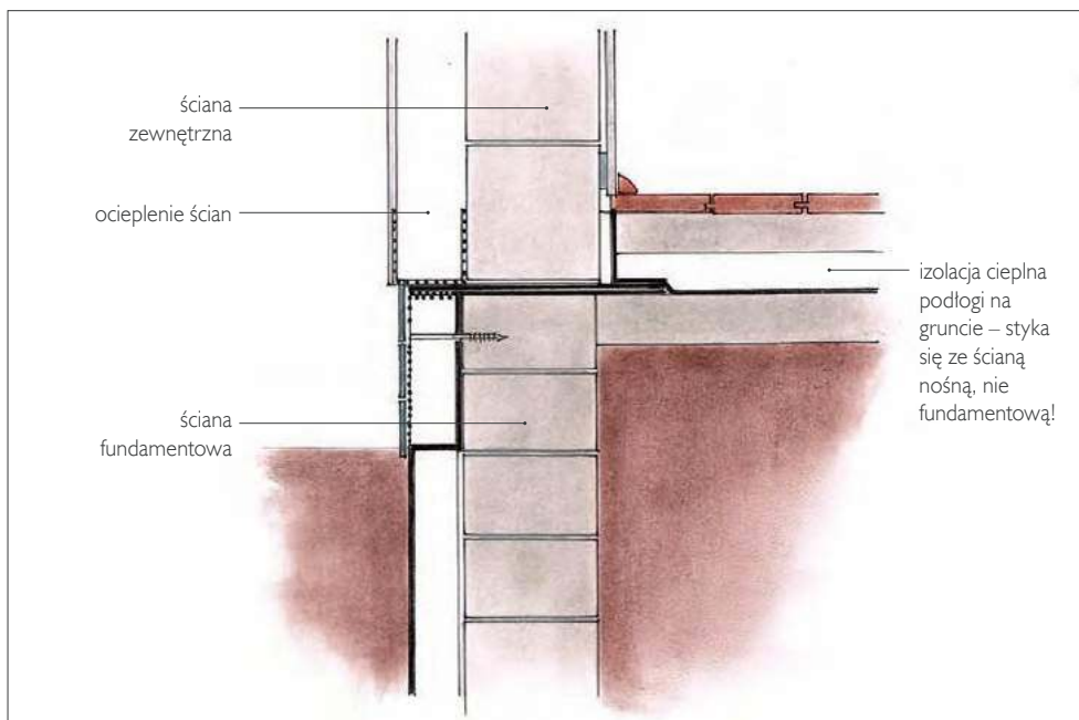
📌 Prawidłowe połączenie izolacji cieplnej ściany fundamentowej, zewnętrznej i podłogi na gruncie.
