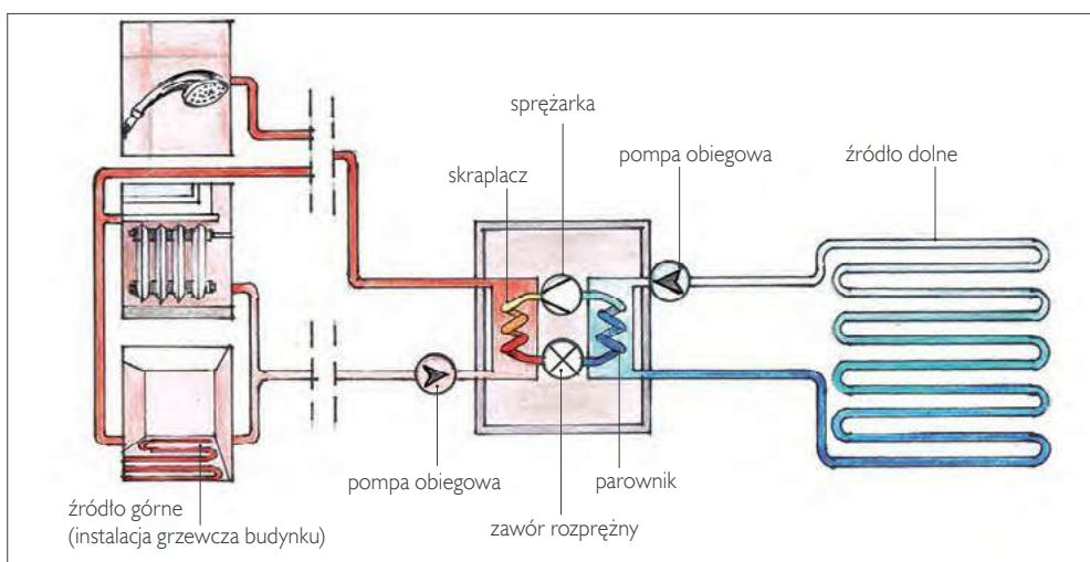
🔧 Zasada działania pompy ciepła.
