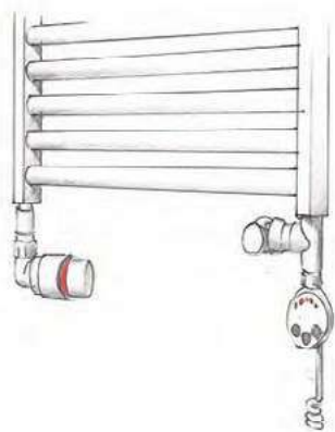
Rys. 1 Typowa drabinka o symetrycznym kształcie ma 2 przyłącza u dołu. Najczęściej grzałkę podłącza się poprzez dodatkowy trójnik założony na powrocie.
