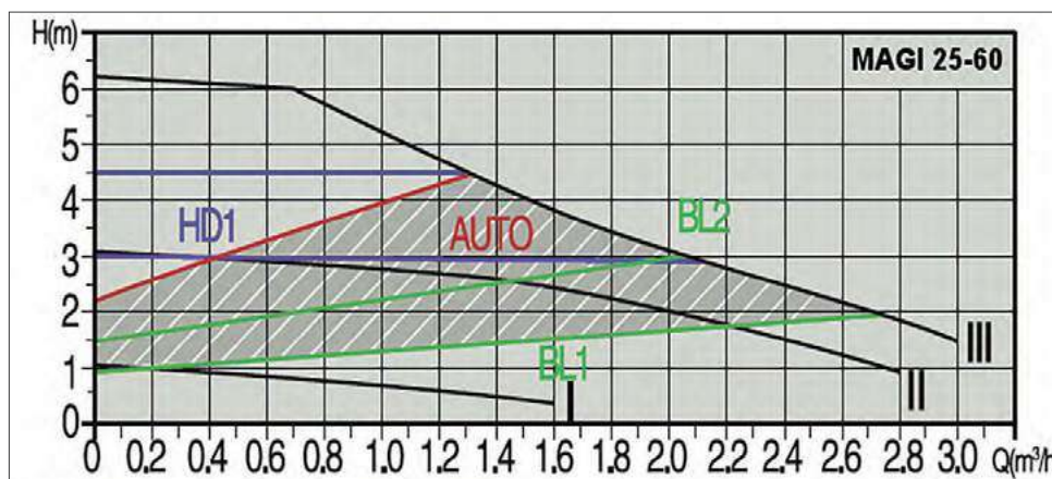
Charakterystyka pompy o takim samym maksymalnym przepływie, ale większej wysokości podnoszenia (6 m). Warto zauważyć, że zakresy pracy częściowo się pokrywają, a bieg pierwszy (I) jest identyczny. IBO (DAMBAT)
