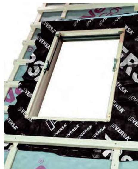
Specjalnym typem okien połaciowych są wyłazy dachowe, które montuje się zazwyczaj w pobliżu komina. Na zdjęciu model zintegrowany z kołnierzem z membrany paroprzepuszczalnej, umożliwiającej szczelne połączenie izolacji przeciwwilgociowej stolarki z membraną paroprzepuszczalną połaci dachu. OKPOL
