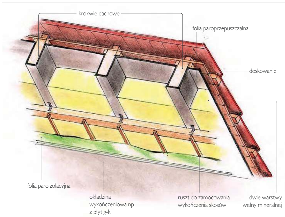
❶ Ocieplenie dachu skośnego wełną mineralną.
