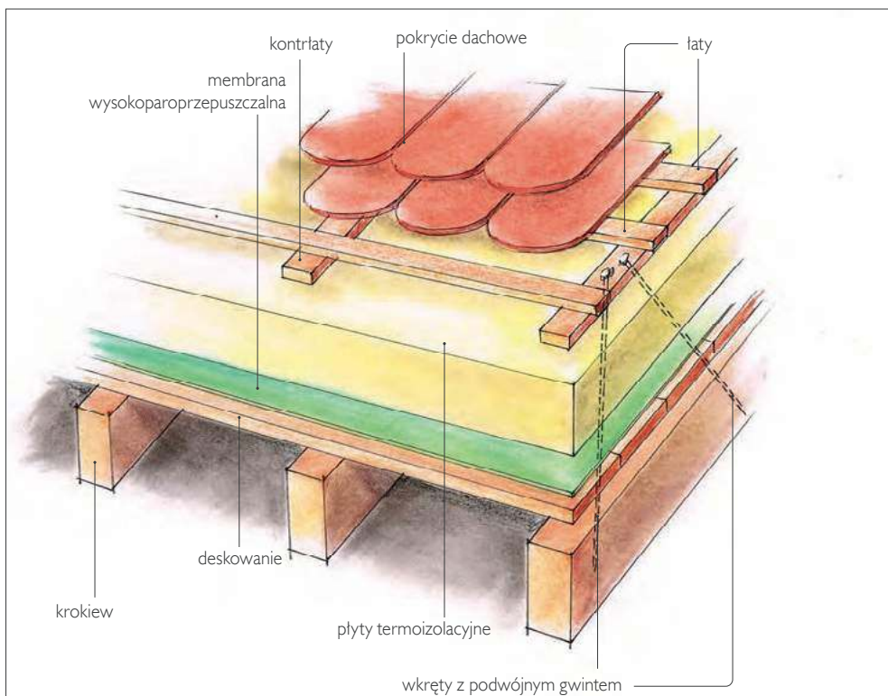
❷ Schemat ocieplenia nastrogowego.
