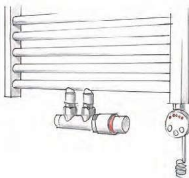
Rys. 2 Podłączenie centralne dolne, tzw. D50. Sprawdźmy po której stronie producent dopuszcza montaż grzałki.
