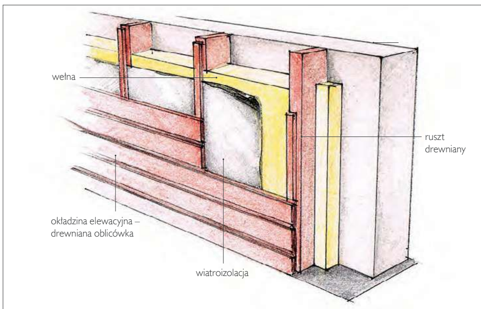
Ściana dwuwarstwowa ocieplona metodą lekką suchą.
