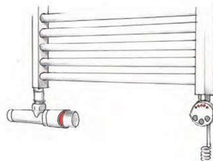
Rys. 3 Podłączenie dolne przez specjalny zawór rurowy. Zasilanie i powrót zajmują wówczas tylko jeden króciec grzejnika.
