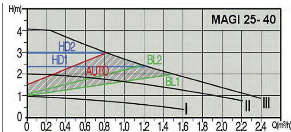
Wykres charakterystyk pompy elektronicznej. I, II, III to odpowiedniki zwykłych biegów – stała prędkość obrotowa). BL1, BL2 – utrzymanie stałego przepływu, zaś HD1, HD2 to stała wysokość podnoszenia. W funkcji Auto pompa sama dobiera optymalne parametry pracy. IBO (DAMBAT)
