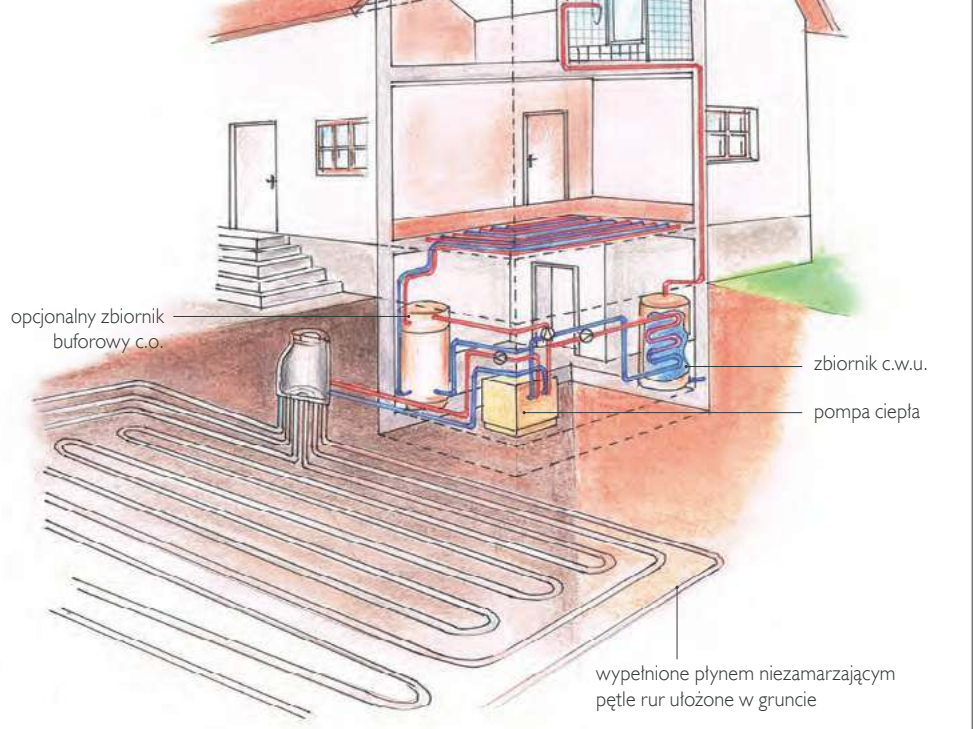
Gruntowy kolektor poziomy.
