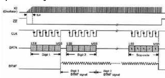
Rys. 9. Stany logiczne generatora w układzie HT9200
