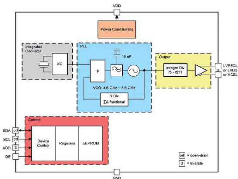
Rys. 1. Schemat blokowy LMK61E2
