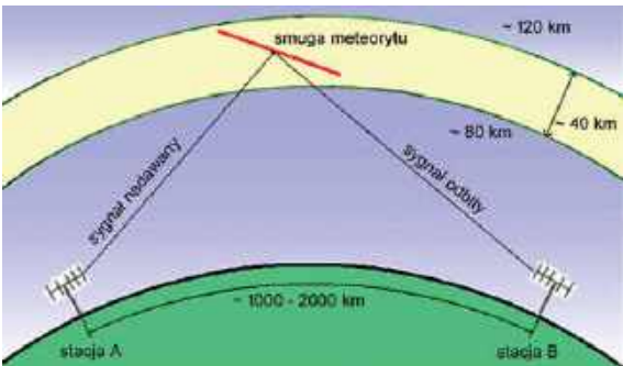
Rys. 5. Łączność za pośrednictwem odbić od zjonizowanych smug meteoroidów (MS)
