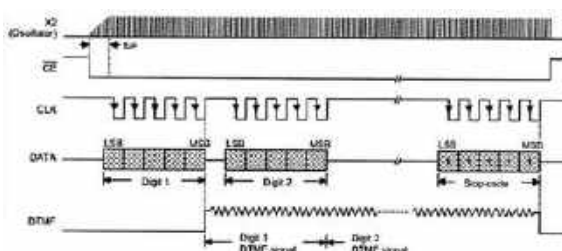
Rys. 9. Stany logiczne generatora w układzie HT9200
