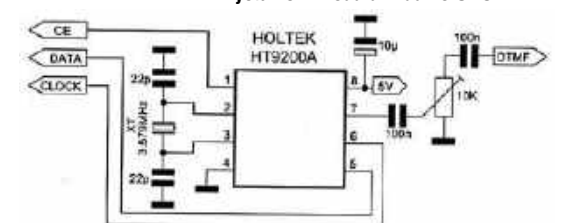
Rys. 8. Schemat generatora tonu na układzie HT9200
