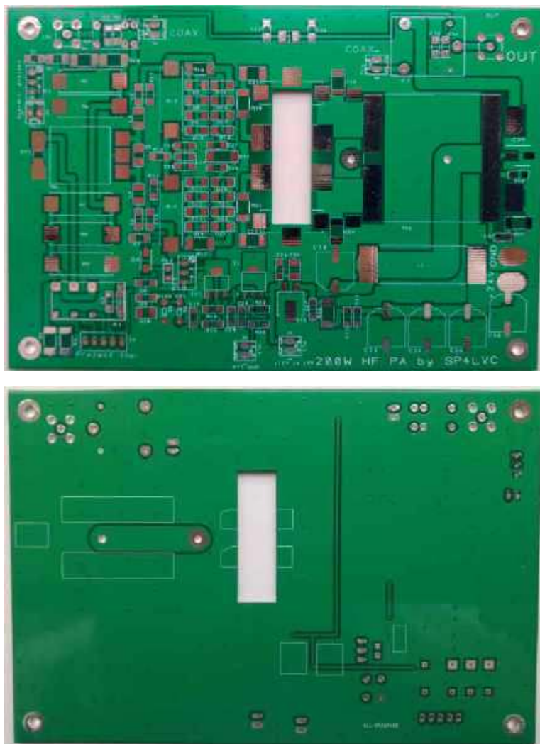
Dwustronna płytki wzmacniacza
