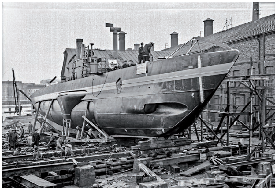
▲ Czwartym okrętem podwodnym był Saukko (Sa 241) o wyporności nawodnej 99 ton i podwodnej 114 ton. Okręt został zbudowany z myślą o działaniach na Jeziorze Ładoga. Z boku doskonale widoczne są zewnętrzne zbiorniki balastowe. Okręt uzbrojony był w dwie torpedy kalibru 450 mm (wyrzutnie dziobowe) oraz sześć min.
