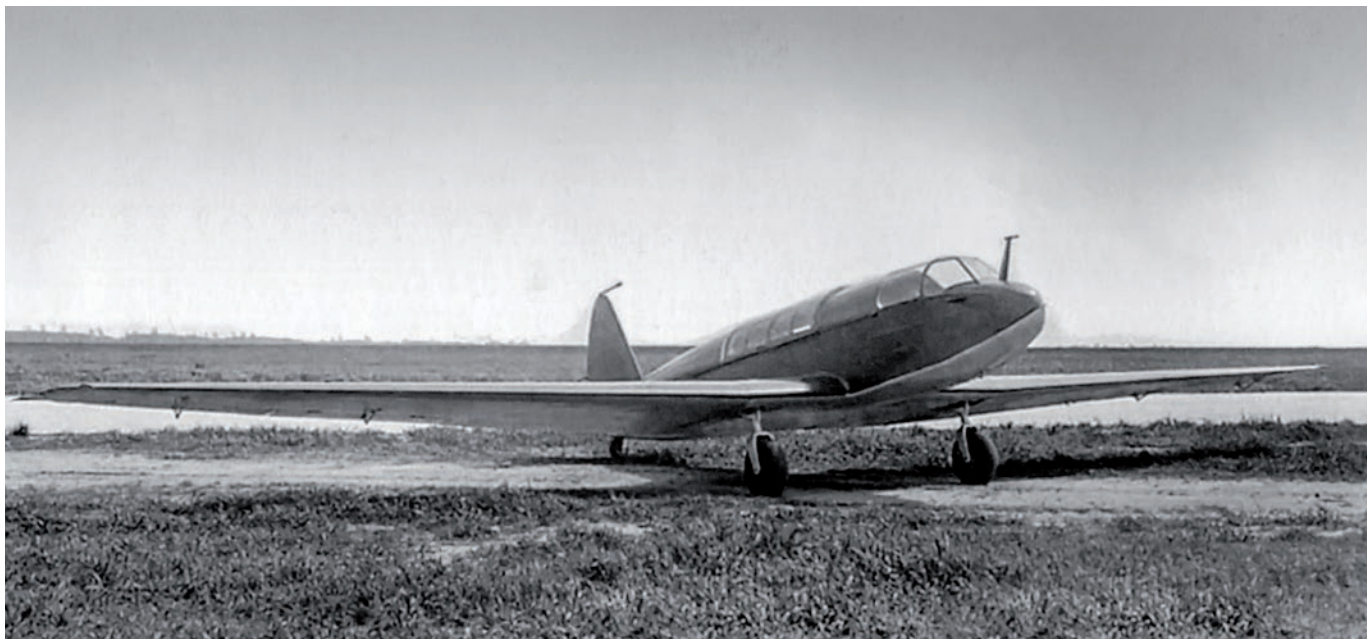
▲ Szybowiec Sokoł na lotnisku w ujęciu 3/4 od przodu. Widać konstrukcję podwozia. Przed kabiną na słupku dysza prędkościomierza. Na szczycie steru kierunku wyważenie. Uwagę zwracają opływowe kształty kadłuba i płat o znacznym wydłużeniu.
