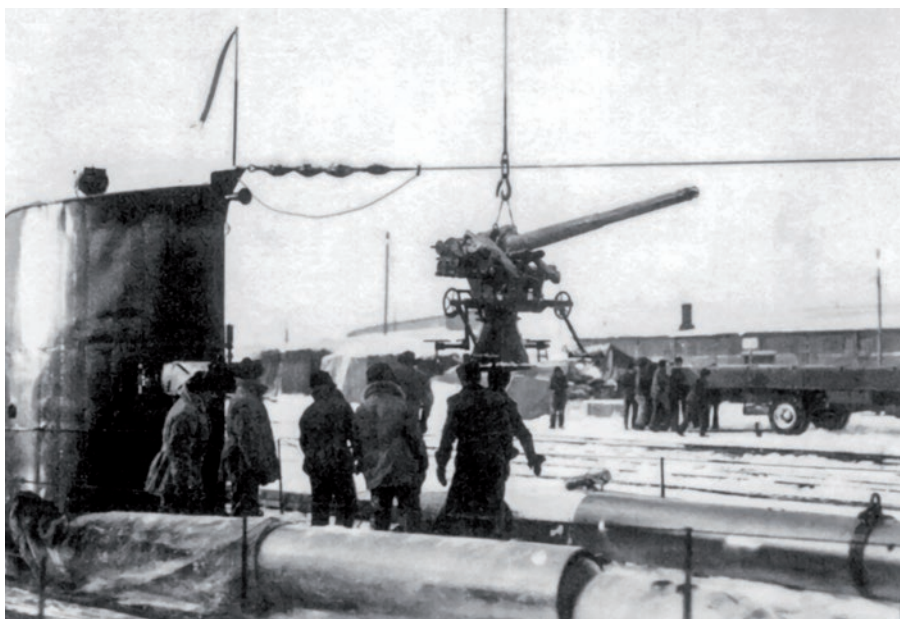
▲ Okręty podwodne Vetehinen , Vesihisi i Iku-Turso uzbrojone były także w półautomatyczną armatę kalibru 76,2 mm ULK firmy Bofors (w Finlandii oznaczoną jako 76/48 28 LT), zamontowaną na okrętach w latach 1930–1931. Można było z niej prowadzić ogień do celów morskich i powietrznych. W trakcie wojny zimowej działa zostały zdemontowane.
