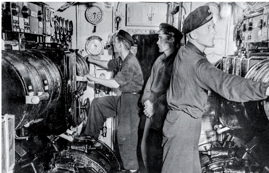
▲ Przedział silników elektrycznych na okręcie podwodnym Vetehinen (CV-702). Okręty wyposażono w dwa szwajcarskie silniki Brown-Boveri o mocy 360 KM przy 420 obr./min.
