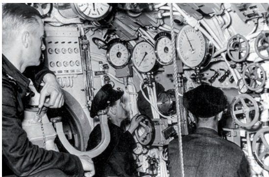
▲ Centrala okrętu podwodnego Vesihisi (CV-703). Widoczne stanowisko obsługi sterów głębokości.
