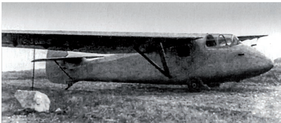
◀ Mały szybowiec G nr 4 z pierwszą wersją osłony kabiny. Na boku widać okno kabiny desantu. Na przedniej części kadłuba widać przyrządy pomiarowe. Szybowiec jest „zakotwiczony” do solidnego bloku betonowego. Uwagę zwraca staranne opracowanie aerodynamiki płatowca.
