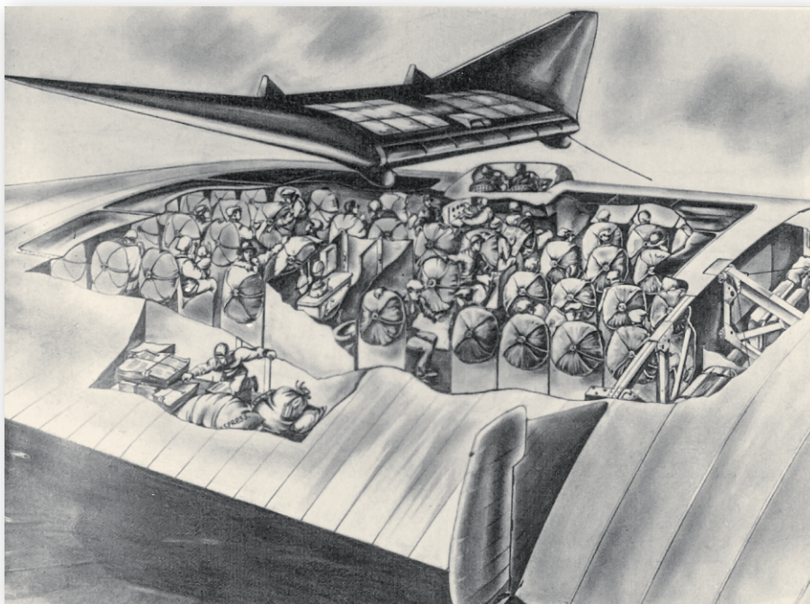
▲ Wariant szybowca występujący pod oznaczeniem G-64. W tym przypadku jest więcej okien nad przedziałem transportowym, inna jest osłona kabiny pilotów a usterzenie ma mniejszą powierzchnię. Część ilustracji przedstawia rozmieszczenie desantu wewnątrz płata. Jak widać część żołnierzy miała podróżować przy krawędzi spływu.
