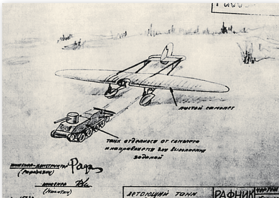
▲ Oryginalny rysunek dołączony do projektu latającego czołgu. Przedstawia chwilę po rozłączeniu pojazdu z płatowcem. Śmigło napędzające jest ustawione w pozycji horyzontalnej. Projekt nosił nazwę „Rafnik”.
