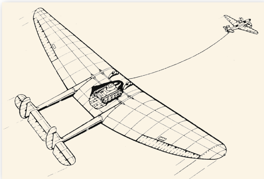
▲ Projekt olbrzymiego szybowca G-67 w układzie latającego skrzydła z dwiema belkami ogonowymi połączonymi usterzeniem. Standardowy czołg BT miał być transportowany wewnątrz płata. Widać dwie oddzielne kabiny pilota. Samolot holujący przypomina DB-3 będący w tym czasie jeszcze w fazie projektu. Porównanie gabarytów daje pojęcie o rozmiarach G-67.
