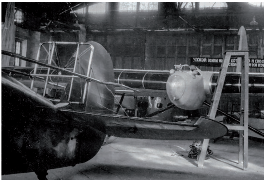
▲ Widok na przód szybowca G-31 stojącego w hangarze. Widać wejścia do komór ładunkowych w krawędzi natarcia płata. Na pierwszym planie stoi samolot holujący R-5 z dobrze widoczną ramą chroniącą usterzenie. Po lewej stronie tej ramy znajduje się sztywna końcówka liny holowniczej.
