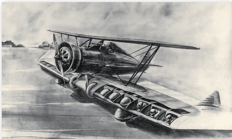
▲ Dołączona do projektu artystyczna wizja „zestawu desantowego” G-53 złożonego z samolotu myśliwskiego I-5 przenoszącego latające skrzydło transportowe. Na rysunku widać żołnierzy desantu w trzech zewnętrznych komorach transportowych. W pozostałych znajdują się jakieś ładunki.
