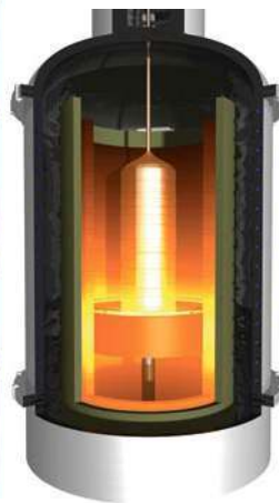
Grafika przedstawiająca przemysłowy proces Czochralskiego służący do uprawy kryształów krzemu
