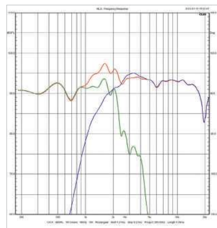
rys. 3. Charakterystyki przetwornika nisko-średnionowego i wysokotonowego i ich suma.
