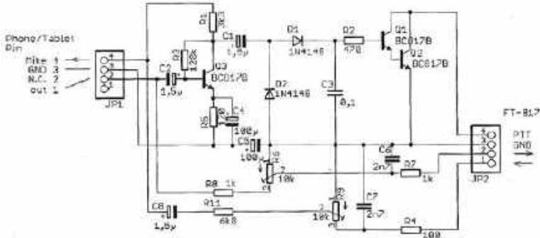
Rys. 7. Schemat prostego interfejsu komputer – radiostacja
