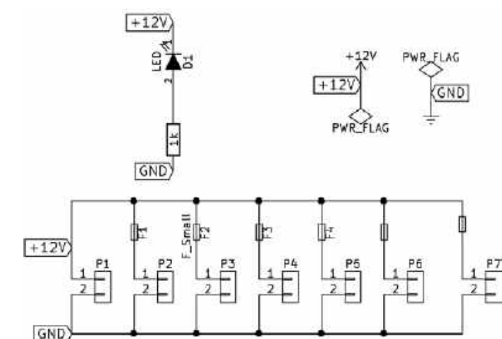
Rys. 16. Schemat ideowy rozgałęźnika zasilania
