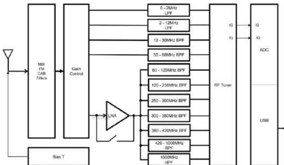
Rys. 3. Schemat blokowy RSP1A
