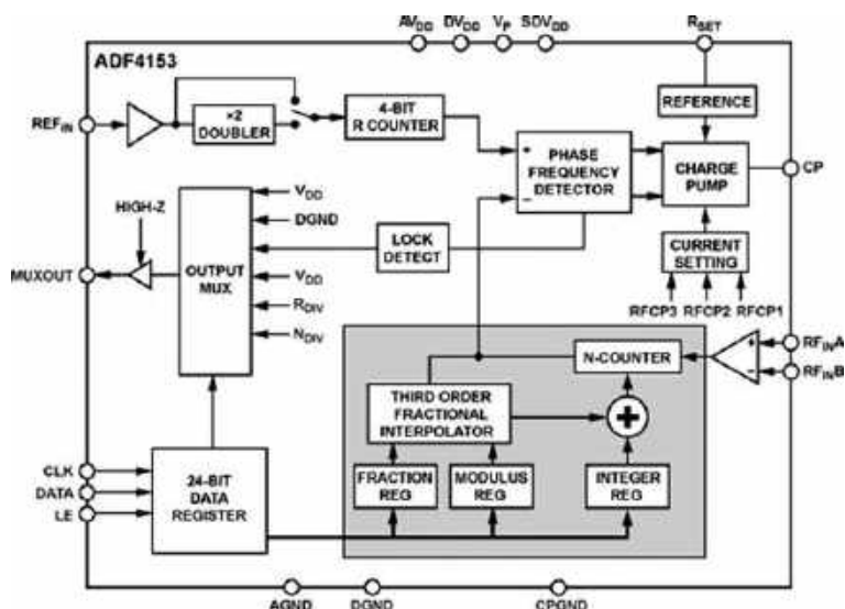
Rys. 2. Schemat blokowy srtruktury ADF4153
