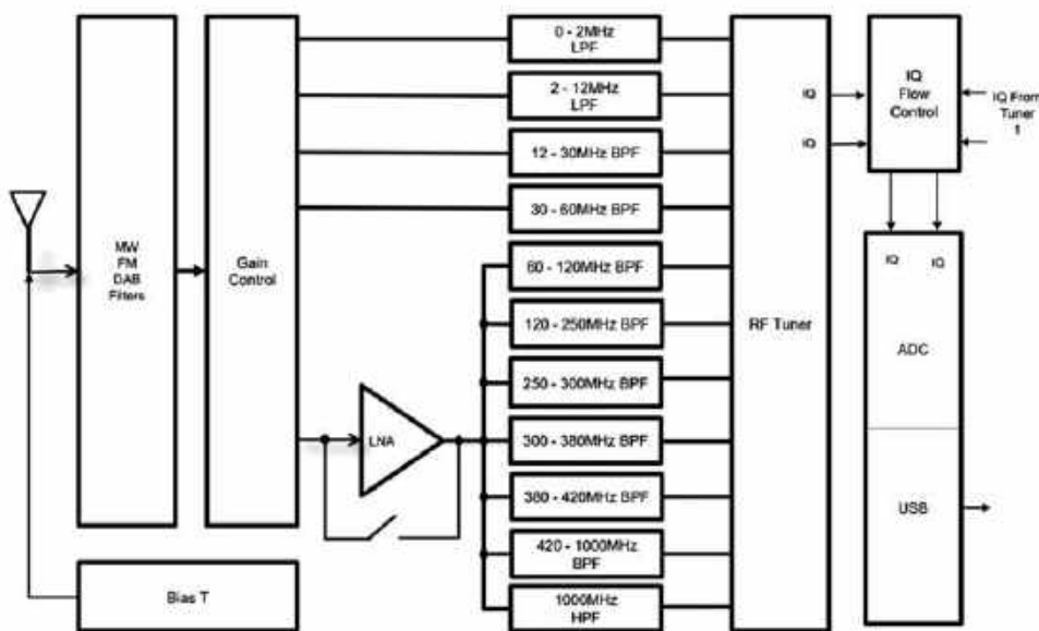
Rys. 5. Schemat blokowy toru odbiorczego Tuner 2
