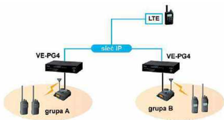
Rys. 3. Przykład połączenia sieci radiowych w różnych lokalizacjach przez bramkę VE-PG4
