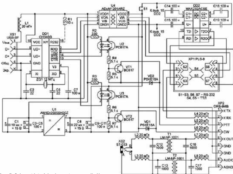
Rys. 5. Schemat interfejsu komputerowego dla Yaesu
