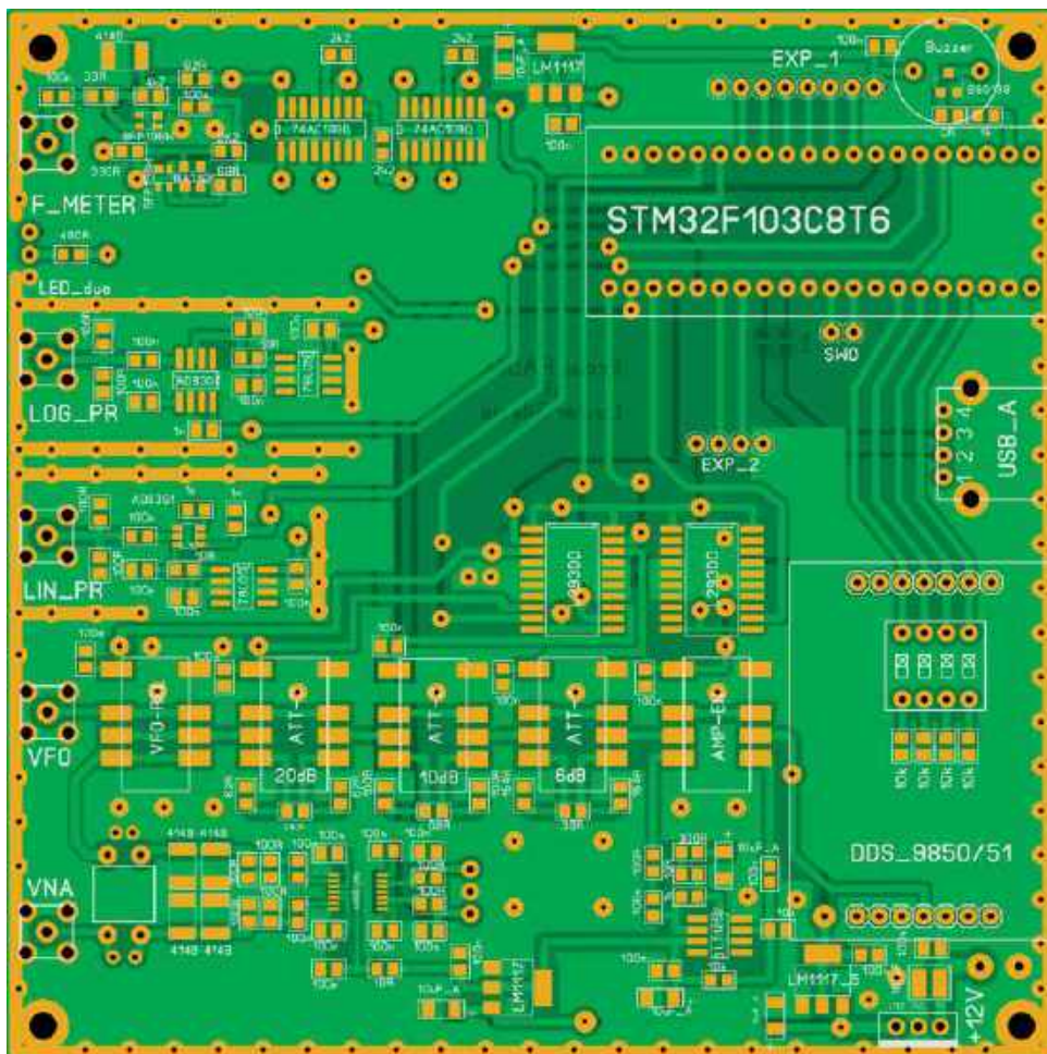
Rys. 19. Nowa płytka PCB radiotestera
