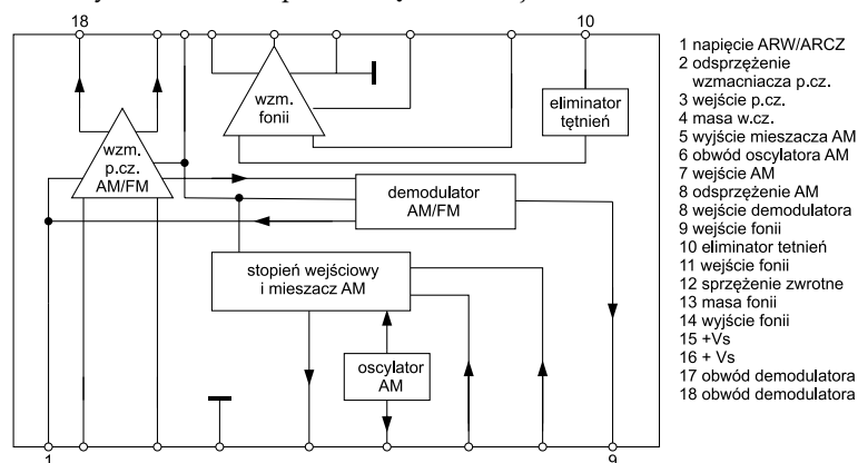
Rys. 3. Rozkład wyprowadzeń układu U-418
