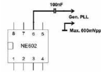
Rys. 3. Sposób podłączenia syntezy częstotliwości
