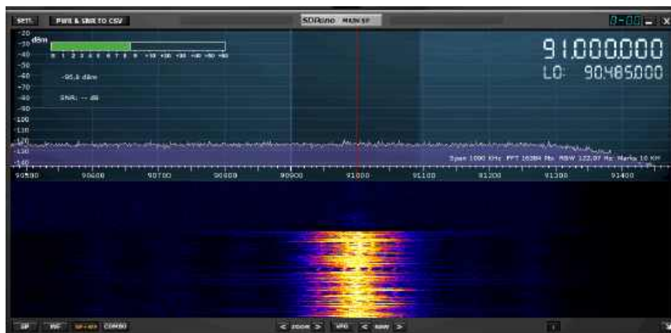
Rys. 10. Filtr notch dla pasma UKF FM
