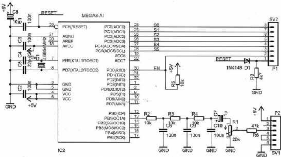
Rys. 9. Schemat enkodera CTCSS
