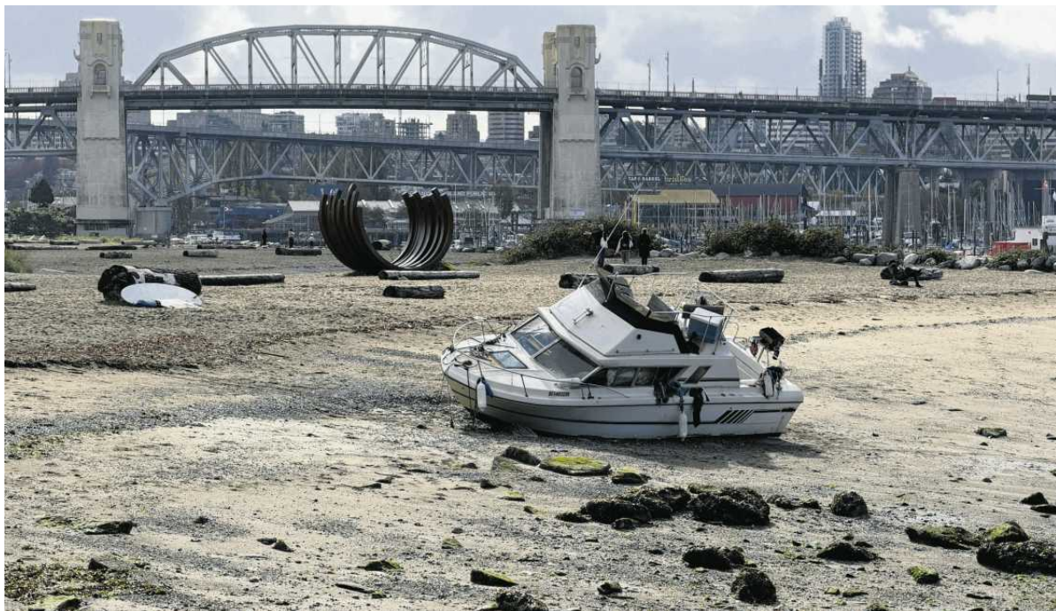
26 września 2026 roku, Vancouver, Kolumbia Brytyjska. Łódź wyrzucona na plażę Sunset Beach podczas wichury, która przeszła nad okolicą dzień wcześniej.
