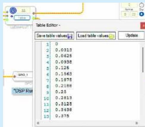
Rysunek 20. Tablica sterująca regulatorem poziomu
