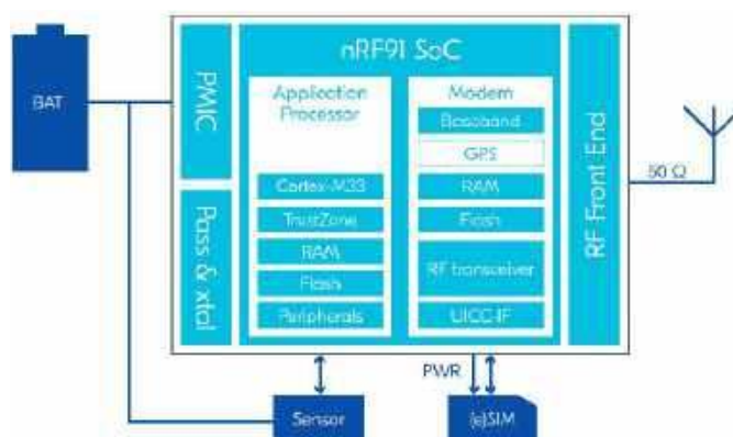
Rysunek 4. Uproszczony schemat aplikacyjny układu nRF9160 ( https://t.ly/8NVo- )
