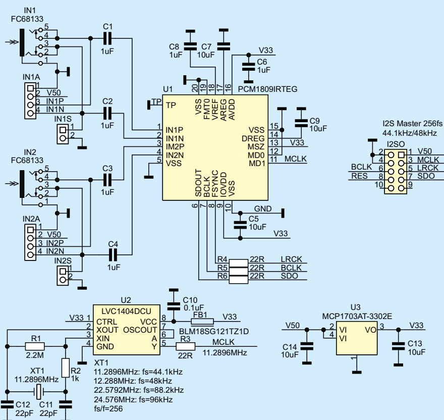
Rysunek 2. Schemat ideowy modułu rozszerzenia DSP1701A_AD_PCM1809
