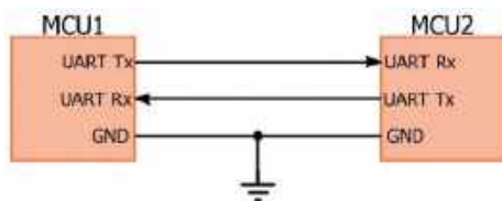
Rysunek 6. Podstawowa struktura łącza UART ( https://t.ly/XPHm )
