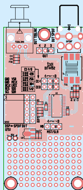
Rysunek 13. Rozmieszczenie elementów DSP1701A_SPDIF_OUT_DIT4192
