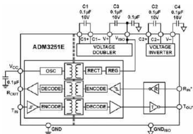
Rysunek 25. Schemat budowy izolowanego transceivera RS-232 typu ADM3251E ( https://t.ly/rj3gc )
