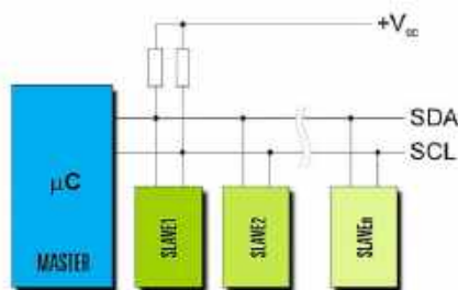
Rysunek 10. Schemat typowej magistrali I 2 C ( https://t.ly/6KuzT )
