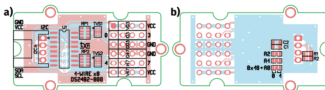
Rysunek 3. Rozmieszczenie elementów na PCB modułu (a – strona TOP, b – strona BOTTOM)
