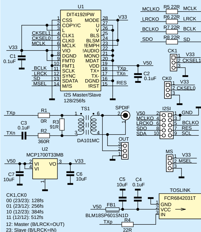
Rysunek 12. Schemat ideowy modułu DSP1701A_SPDIF_OUT_DIT4192
