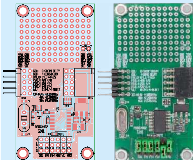
Rysunek 15. Rozmieszczenie elementów DSP1701A_ASRC4192
