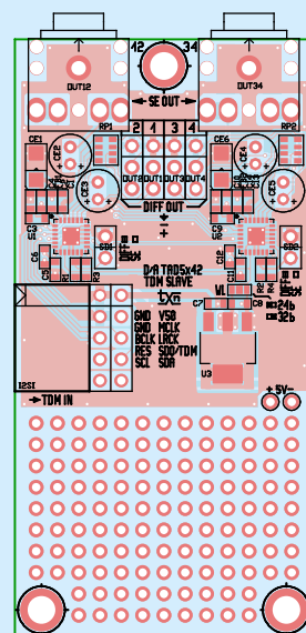
Rysunek 9. Rozmieszczenie elementów DSP1701A_DACTDM_TAD5142
