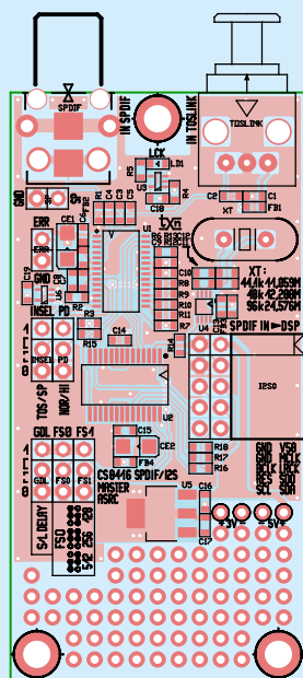
Rysunek 11. Rozmieszczenie elementów DSP1701A_SPDIF_IN_ARSC
