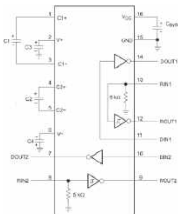
Rysunek 24. Typowa aplikacja układu TRSF3232 ( https://t.ly/DGD2F )
