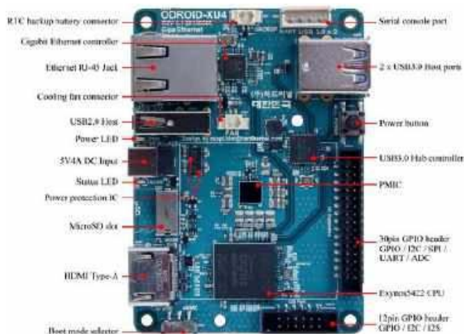
Fotografia 2. Płytkę nowoczesnego minikomputera Odroid XU4 z zaznaczonymi najważniejszymi komponentami. W górnej części płytki, obok interfejsów USB 3.0, umieszczono klasyczny interfejs UART oznaczony jako Serial Console Port ( https://t.ly/zDj5b )
