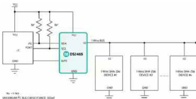
Rysunek 5. Uproszczony schemat systemu z układem DS2465 ( https://t.ly/DSFLK )
