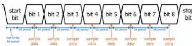
Rysunek 9. Synchronizacja i próbkowanie ciągu bitów w odbiorniku UART ( https://t.ly/8kOYP )
