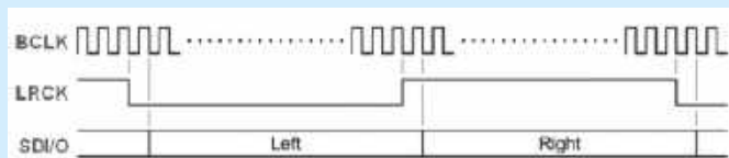
Rysunek 3. Ramka formatu I²S
