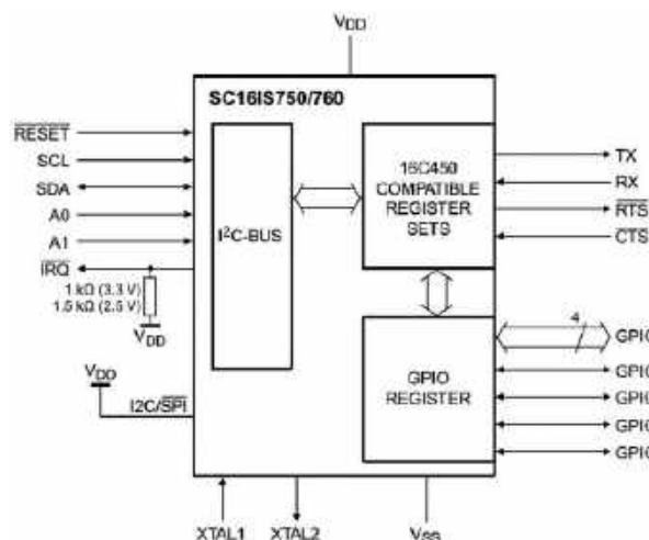
Rysunek 15. Uproszczony schemat blokowy układu SC16IS750/760 ( https://t.ly/Z36I5 )
