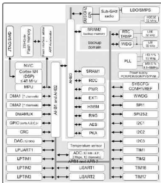
Rysunek 5. Schemat blokowy mikrokontrolera z serii STM32WLE5 ( https://t.ly/Bf6Z_ )
