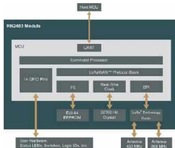
Rysunek 7. Uproszczony schemat blokowy modułu RN2483 ( https://t.ly/Ybg90 )
