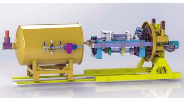
Rysunek spektrografu NIRPS, zamontowanego na jednym z teleskopów Obserwatorium La Silla w Chile
