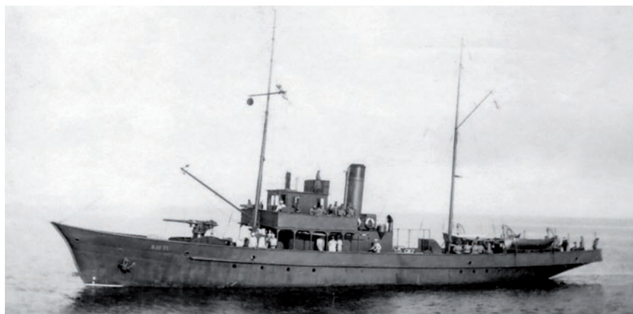
◀ W 1918 roku w stoczni Ahlström Oy w Varkaus zbudowano jeden z czterech trałowców bazowych typu Udamnik . Okręt miał 220 ton wyporności i był uzbrojony w jedną armatę wz.1906 kalibru 75 mm. Otrzymał nazwę Fortra . Okręt został przetransportowany w częściach ze stoczni kanałem Saimańskim do Wyborga, gdzie otrzymał nową nazwę Rautu . Jednostka została kupiona od stoczni dopiero w kwietniu 1920 roku. Pozostawała w służbie do 1948 roku. W 1952 roku została skreślona ze stanu i sprzedana na złom.
