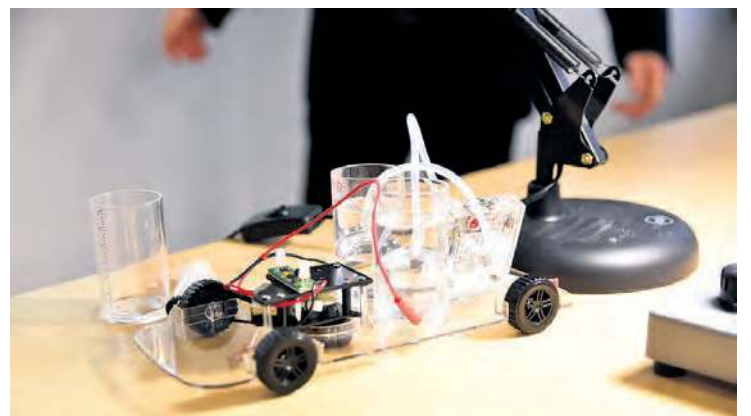
Model pojazdu napędzanego energią ze słonej wody.
