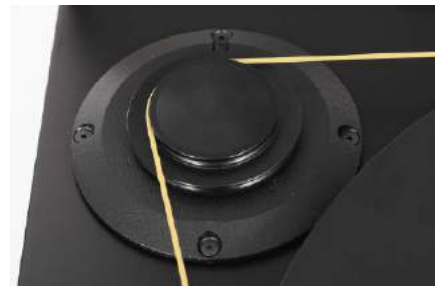
Silnik jest osadzony na elastycznej podstawie, zmiana prędkości obrotowej wymaga przełożenia paska na sąsiednie koło.
