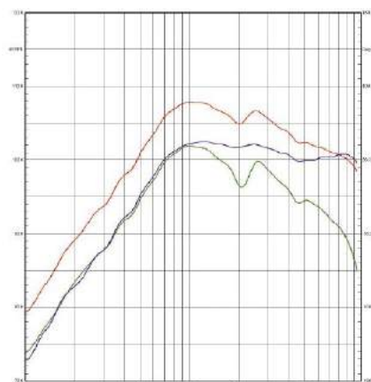
Rys. 4c. Charakterystyki sekcji niskotonowej, nisko-średniotonowej i charakterystyka zespołu – obydwa bas-refleksy zamknięte (poniżej 1 kHz, pomiar w polu bliskim).
