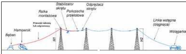
Grafika obrazująca sposób montażu przewodów
