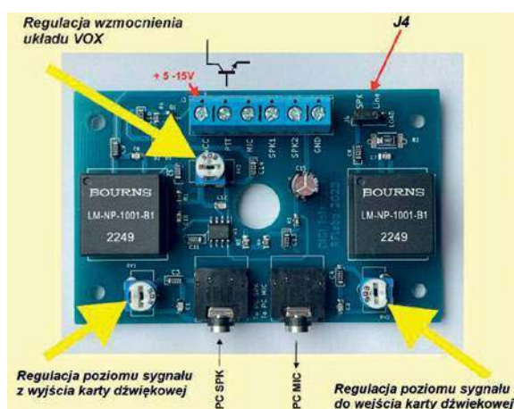
Rys. 1 Widok zmontowanego urządzenia z opisami złączy i regulacji
