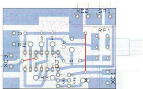
Rys. 7. Płytką drukowaną wykrywacza metali
