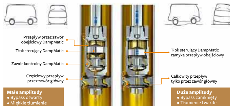
Schemat działania układu DampMatic II
