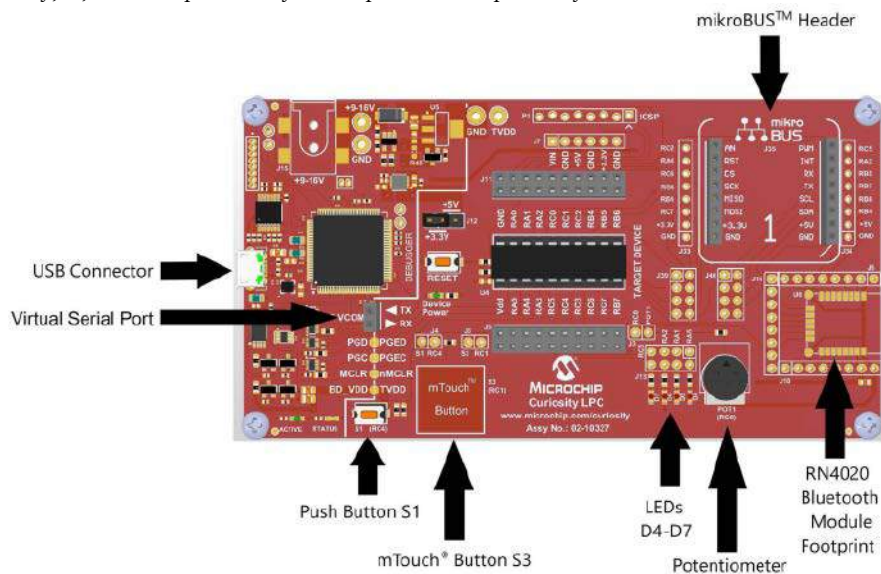
Rysunek 1. Rozmieszczenie podstawowych komponentów na płytce (wersja płytki – Rev 4)
