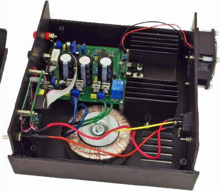
Fotografia 6. Wygląd wnętrza zasilacza pokazujący podzespoły osadzone na płycie tylnej i płycie przedniej oraz sposób montażu podzespołów na spodzie obudowy
