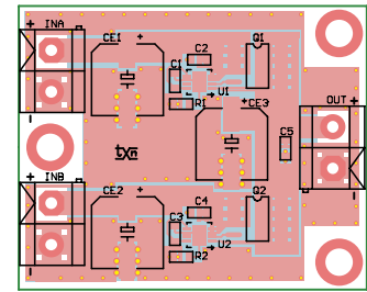
Rysunek 3. Schemat płytki PCB
