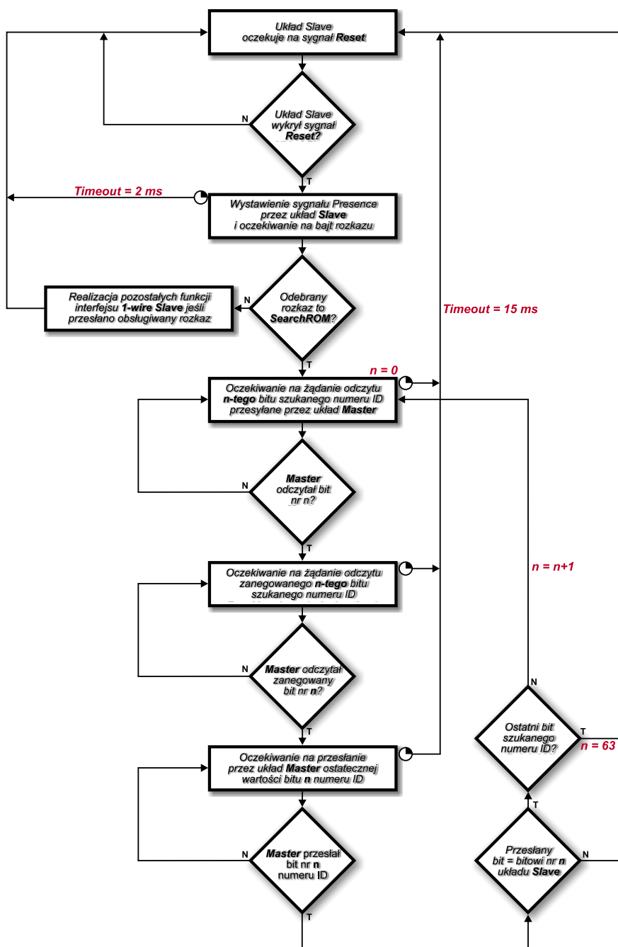
Rysunek 5. Sekwencja sygnałów sterujących obrazująca mechanizm znajdowania numerów ID układów Slave (z punktu widzenia tychże układów)
