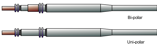
Rysunek 13. Porównanie konstrukcji złączy IS-1 Bi (na górze) i IS-1 Uni (na dole). Czerwone elementy oznaczają pola stykowe, niebieskie – uszczelnienia, pozostała część to izolacja przewodu oraz złącza (https://t.ly/nwUq)
