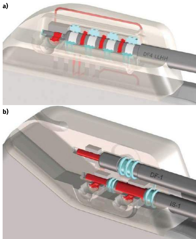
Rysunek 16. Szczegóły konstrukcyjne gniazd DF-4, DF-1 oraz IS-1. Niebieskim kolorem oznaczono uszczelnienia: w przypadku DF-4 (rysunek A) są one umieszczone bezpośrednio w gnieździe (bloku złącz), podczas gdy wtyki DF-1 i IS-1 zapewniają własne uszczelnienia, współpracujące jedynie z odpowiednio wyprofilowanymi otworami w bloku złączy (rysunek B). Źródło: https://t.ly/JApn
