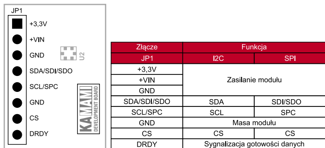
Rysunek 13. Moduł czujnika wilgotności KAMod HTS221
