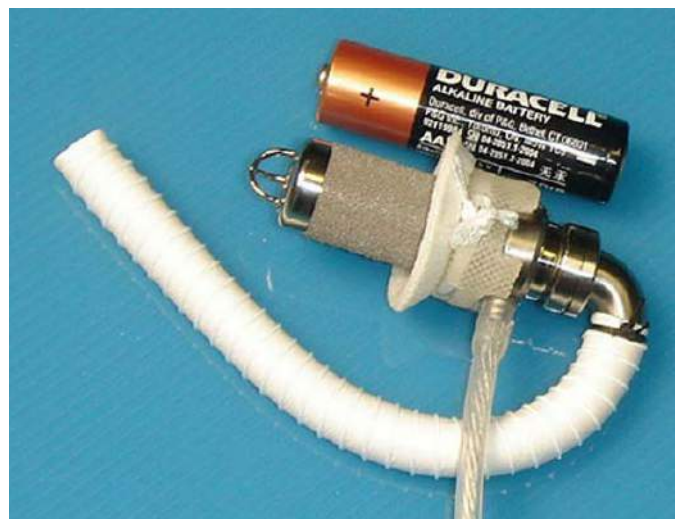
Fotografia 24. Jarvik 2015 – jeden ze współcześnie stosowanych modeli pomp do wspomagania lewej komory serca (LVAD). Niewielkie urządzenie jest przeznaczone dla, małych dzieci, stąd tak kompaktowe wymiary całości (porównanie z baterią typu AA). Źródło: https://t.ly/gylr
