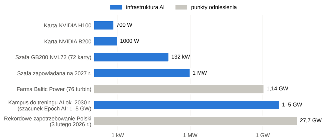
Rysunek 8. Od karty graficznej do kampusu treningowego – moc elektryczna infrastruktury AI na tle polskich punktów odniesienia. Skala logarytmiczna. Źródła: NVIDIA (karty H100 i B200, zapowiedź szaf 1 MW), Schneider Electric (szafa NVL72), Epoch AI (2024, szacunek mocy największego kampusu treningowego ok. 2030 r.), Orlen (Baltic Power), PSE (rekord zapotrzebowania)
