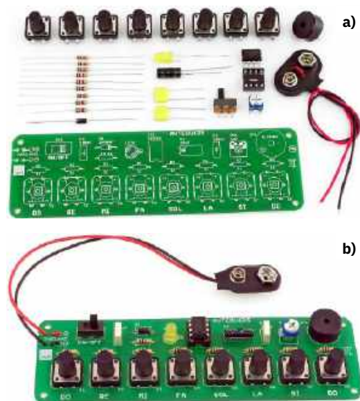
Fotografia 1. Minipianino (kod AVTEDU635): a) zestaw do samodzielnego montażu, b) zmontowany układ
