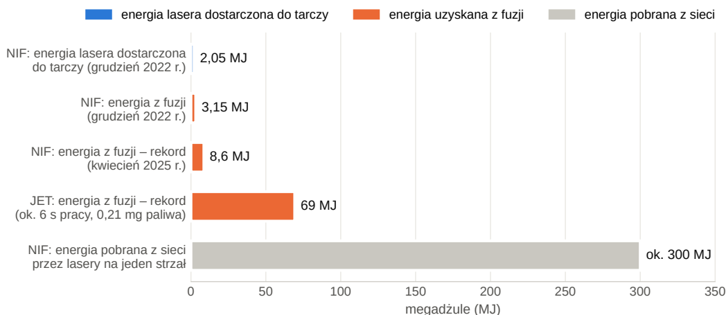
Rysunek 19. Bilans energii w rekordowych eksperymentach fuzyjnych. Energia pobrana z sieci przez lasery NIF (ok. 300 MJ) dotyczy strzału z grudnia 2022 r. Źródła: Lawrence Livermore National Laboratory; Optica, Optics & Photonics News (2022); EUROfusion (JET)
