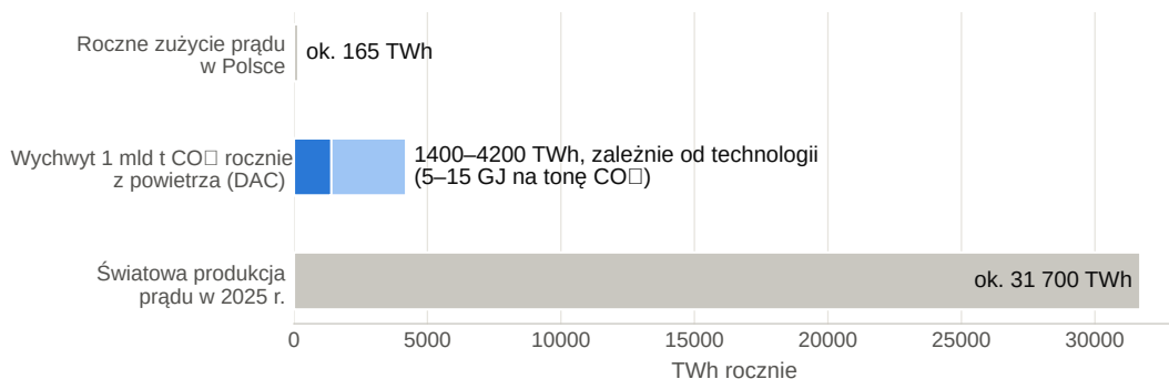
Rysunek 18. Ile energii potrzebowałby wychwył miliarda ton CO 2 rocznie bezpośrednio z powietrza – w porównaniu z rocznym zużyciem prądu w Polsce i światową produkcją energii elektrycznej. Ciemniejszy fragment słupka: wariant najoszczędniejszy (5 GJ na tonę), jaśniejszy: wariant najbardziej energochłonny (15 GJ na tonę). Źródła: Belfer Center, Harvard (energochłonność DAC); Ember, Global Electricity Review 2026 (produkcja światowa – przeliczenie redakcji); KPEiK (Polska)
