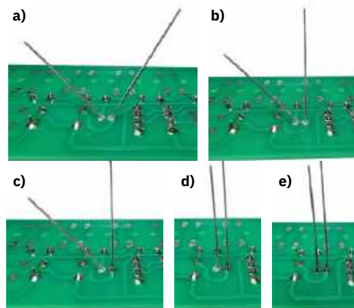
Fotografia 9. Zalecany sposób montażu diody LED, który umożliwi jej łatwą wymianę w przypadku uszkodzenia lub omyłkowego zamontowania w odwrotnym kierunku: a) rozegnij wyprowadzenia diody LED w taki sposób, by dało się bezpiecznie odwrócić płytkę do góry nogami; b) po ustawieniu płytki na błacie odegnij jedno wyprowadzenie do pionu; c) przylutuj odgięte do pionu wyprowadzenie prostopadłe do płytki; d) ustaw do pionu drugie wyprowadzenie; e) przylutuj je prostopadłe do płytki
