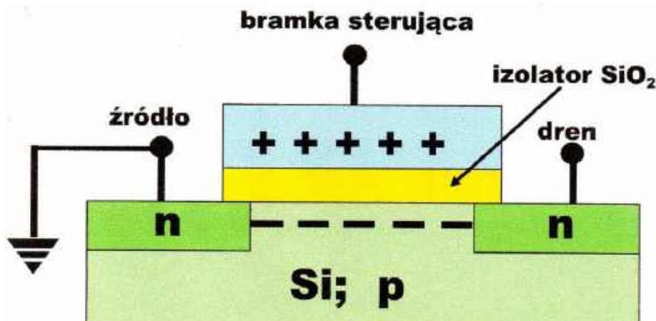
4. Schemat tranzystora MOSFET na podłożu krzemu typu p w stanie przewodzenia
