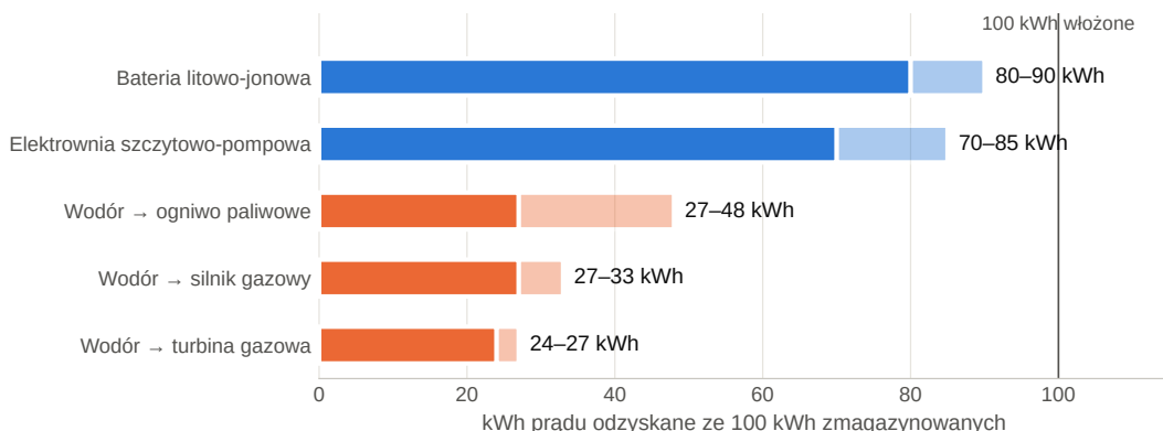
Rysunek 22. Ile prądu odzyskamy ze 100 kWh zmagazynowanych różnymi metodami. Ciemniejsza część słupka: dolna granica przedziału, jaśniejsza: górna. Źródła: Oxford Institute for Energy Studies, „Power-to-Hydrogen-to-Power” (lipiec 2025 r.) – wodór i elektrownie szczytowo-pompowe; EIA (2021) – baterie
