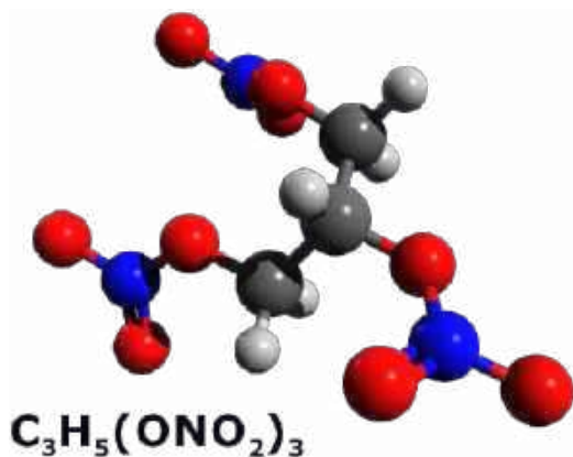
5. Model cząsteczki nitrogliceryny
