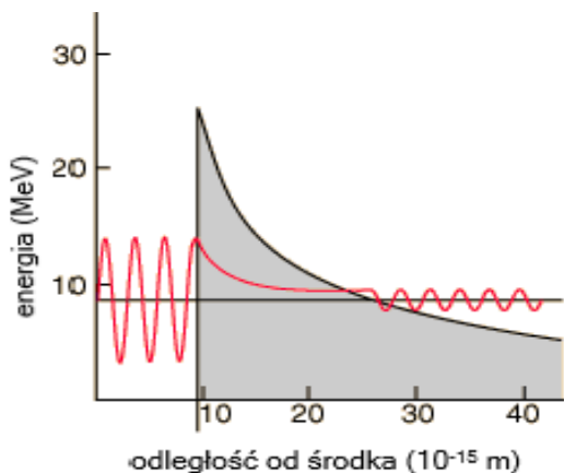
2. Tunelowanie cząstki \alpha poprzez barierę potencjału otaczającą jądro atomu
