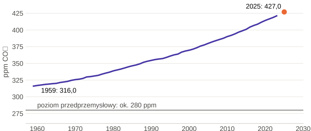
Rysunek 14. Krzywa Keelinga: średnie roczne stężenie dwutlenku węgla w atmosferze mierzone w obserwatorium Mauna Loa na Hawajach. Linia: dane NOAA za lata 1959–2023; punkt: średnia za 2025 r. według zestawienia brytyjskiego Met Office. Źródła: NOAA Global Monitoring Laboratory; Met Office
