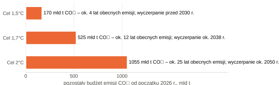
Rysunek 15. Pozostały budżet emisji CO 2 dla trzech granic ocieplenia (przy 50% prawdopodobieństwie ich dotrzymania) i przybliżony rok jego wyczerpania przy utrzymaniu emisji z 2025 r. Źródło: Global Carbon Budget 2025, „Key Targets”; lata wyczerpania – przeliczenie redakcji
