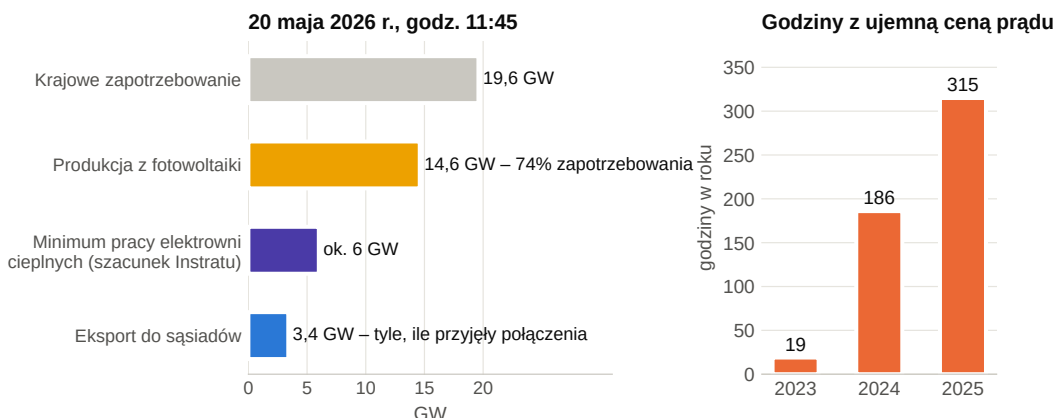
Rysunek 28. Dlaczego w słoneczne południe prądu bywa za dużo. Po lewej: polski system 20 maja 2026 r. o 11:45, gdy fotowoltaika pobiła rekord 14,56 GW i pokrywała 74% krajowego zapotrzebowania; eksport szedł wtedy na maksimum, a w elektrowniach ciepłych i tak musi zostać w ruchu kilka gigawatów. Po prawej: liczba godzin w roku, w których cena energii na giełdzie była ujemna. Źródła: PSE (rekord fotowoltaiki, zapotrzebowanie i eksport – za serwisami wnp.pl i globenergia.pl); Instrat (minimalna praca elektrowni ciepłych); URE (godziny z cenami ujemnymi)
