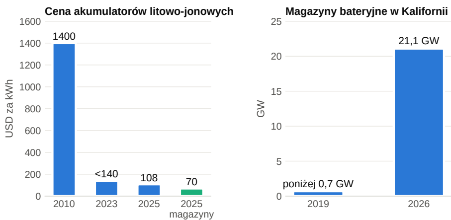
Rysunek 23. Po lewej: średnia cena pakietów akumulatorów litowo-jonowych w USD za kWh pojemności (2010 i 2023 – dane MAE, 2025 – BloombergNEF; słupek „2025 magazyny” to pakiety do magazynów stacjonarnych). Po prawej: moc magazynów bateryjnych w Kalifornii. Źródła: MAE, Batteries and Secure Energy Transitions (2024); BloombergNEF (grudzień 2025 r.); California Energy Commission (sierpień 2026 r.)
