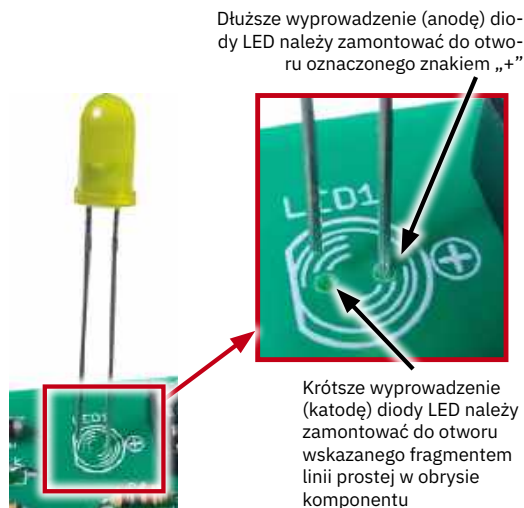
Rysunek 7. Poprawny sposób montażu diody LED w płytce PCB z uwzględnieniem jej polaryzacji. Dłuższe wyprowadzenie (anoda) powinno zostać umieszczone w otworze oznaczonym znakiem „+”, natomiast krótsze wyprowadzenie (katoda) – w otworze oznaczonym linią prostą w obrysie podstawy
