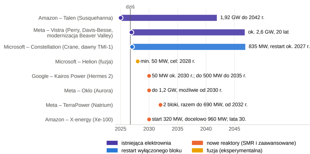
Rysunek 9. Kiedy popłynie prąd z elektrowni jądrowych dla wielkich firm technologicznych. Kółko oznacza planowany początek dostaw, pasek – okres umowy, jeśli został podany. Terminy dla nowych reaktorów i fuzji do deklaracji firm, a nie harmonogramy zatwierdzone przez dozór jądrowy. Źródła: komunikaty Talen, Meta, Constellation, Helion, Kairos Power, Amazon; World Nuclear News (stan na wrzesień 2026 r.)
