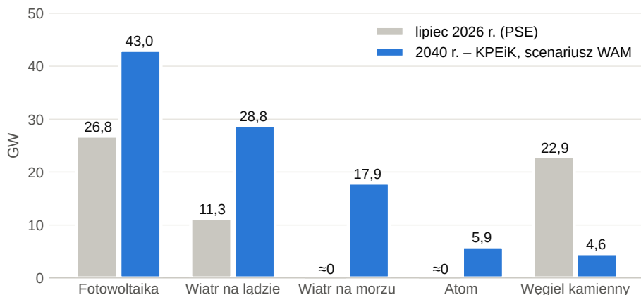
Rysunek 31. Moc zainstalowana wybranych źródeł w Polsce dziś i w 2040 r. według scenariusza WAM Krajowego Planu w dziedzinie Energii i Klimatu. „≈0” – w lipcu 2026 r. pracowała pierwsza część farmy Baltic Power, a elektrownie jądrowe nie istniały. Wartości KPEiK według omówień prasowych (wnp.pl, energetyka24.com). Źródła: PSE (lipiec 2026 r.); KPEiK (2026)
