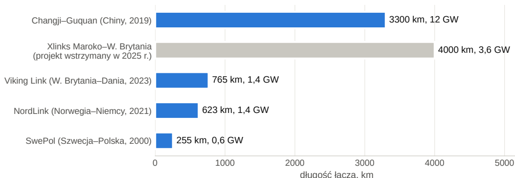
Rysunek 25. Wybrane łącza prądu stałego wysokiego napięcia: długość i moc przesyłowa. Źródła: Hitachi Energy (Changji-Guquan, SwePol); Statnett (NordLink); National Grid (Viking Link); Xlinks i parlament Wielkiej Brytanii (Xlinks)
