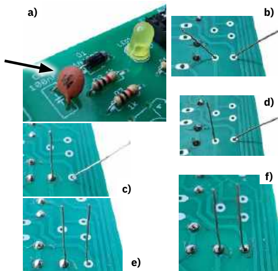
Fotografia 6. Montaż kondensatorów ceramicznych C1 oraz C2: a) kierunek montażu jest obojętny. Na obudowie kondensatora widać napis „104”, informujący o pojemności 10 i 4 zera pikofaradów (100 000 pF), czyli 100 nF; b) po włożeniu kondensatorów do płytki rozegnij lekko ich wyprowadzenia, aby nie wypadły po odwróceniu płytki do góry nogami; c) oprzyj płytkę o blat, a następnie wyprostuj do pionu jedno z wyprowadzeń; d) przylutuj wyprowadzenie pod kątem prostym do płytki; e) wyprostuj do pionu drugie wyprowadzenie; f) przylutuj drugie wyprowadzenie pod kątem prostym do płytki
