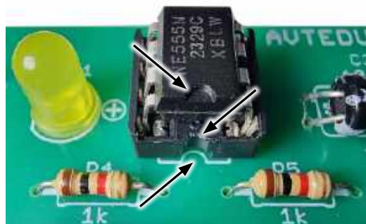
Fotografia 18. Przed zamontowaniem układu scalonego w podstawce należy upewnić się, że znaczniki kierunku montażu – na płycie, w podstawce i na układzie scalonym – znajdują się w tej samej pozycji
