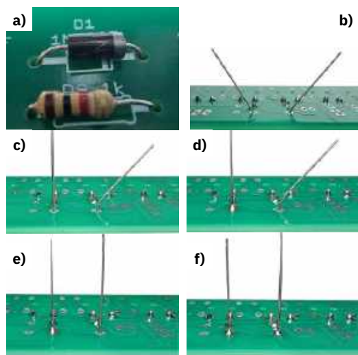
Fotografia 4. Poprawny montaż diody prostowniczej D1 na płytce PCB: a) kierunek pasków na diodzie oraz symbol nadrukowany na płytce musi być zgodny; etapy b), c), d), e) i f) pokazują sposób montażu diody D1, który umożliwia jej łatwą wymianę w przyszłości
