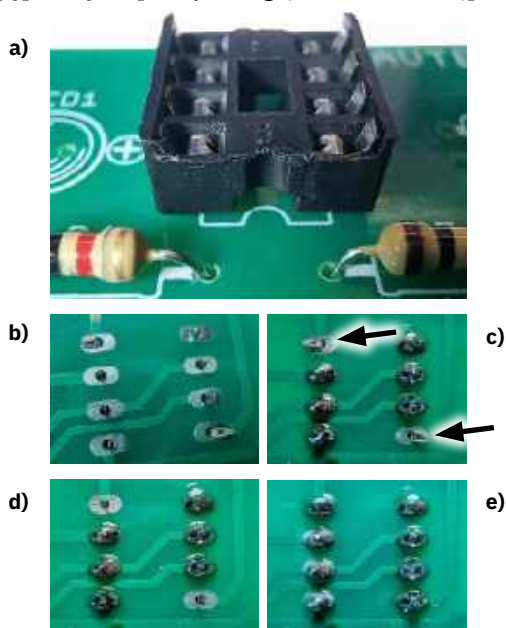
Fotografia 5. a) znacznik kierunku w obudowie podstawki musi być skierowany zgodnie ze wskaźnikiem kierunku nadrukowanym na płytce PCB; b) po włożeniu podstawki do płytki PCB upewnij się, że wszystkie wyprowadzenia przeszły przez otwory, a następnie rozegnij na boki dwa skrajne wyprowadzenia po przekątnej, aby podstawka nie wypadła z płytki po jej odwróceniu; c) przylutuj wszystkie prostopadłe do płytki wyprowadzenia; d) po ich przylutowaniu wyprostuj (ustaw pionowo) dwa pozostałe; e) przylutuj wyprostowane wyprowadzenia do płytki
