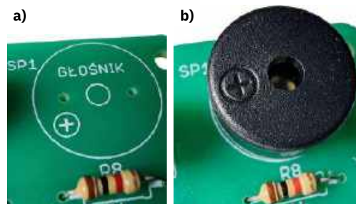
Fotografia 12. a) Oznaczenie polaryzacji na płycie w obrysie pasywnego buzzera; b) oznaczenie polaryzacji na obudowie pasywnego buzzera piezo dołączonego do zestawu; na obu fotografiach pozycję „plusowego” wyprowadzenia komponentu zaznaczono znakiem „+”
