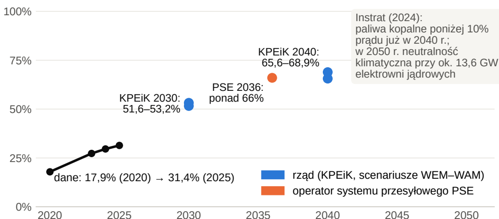
Rysunek 32. Udział odnawialnych źródeł energii w produkcji prądu w Polsce: dane za lata 2020–2025 oraz scenariusze KPEiK (2030, 2040) i PSE (2036). Pionowe odcinki pokazują rozpiętość między scenariuszami WEM i WAM. Instnat (2024) nie podaje udziału OZE w 2050 r.; jego scenariusz zakłada w 2050 r. ok. 13,6 GW elektrowni jądrowych. Źródła: GUS i Forum Energii (dane); KPEiK (2026); PSE, projekt planu rozwoju sieci przesyłowej 2027–2036; Instnat (2024)
