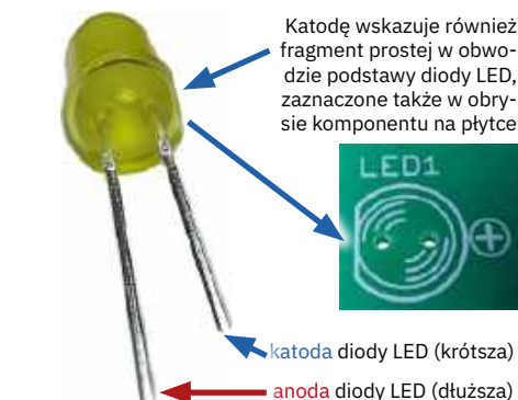
Rysunek 6. Opis wyprowadzeń diody LED („plusowe” wyprowadzenie dłuższe, „minusowe” krótsze)
