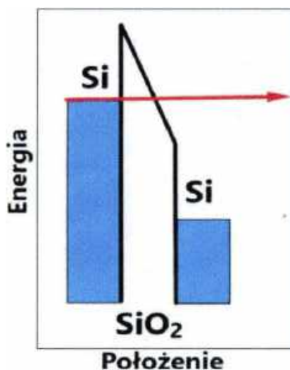
5. Przyłożone duże napięcie modyfikuje barierę potencjału pomiędzy dwiema przewodzącymi warstwami, powodując radykalne zwiększenie prawdopodobieństwa tunelowania
