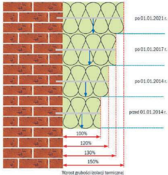
Zmiana grubości izolacji termicznej ścian w okresie 2014-2021 wynikająca ze zmian wymagań w zakresie współczynnika przenikania ciepła U.
